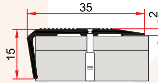
MP 39 0,180 kg/m
