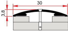
ST 239 B 0,130 kg/m
