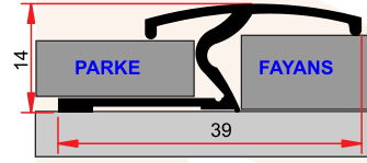
ST 205 0,270 kg/m
