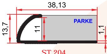
ST 204 0,192 kg/m
