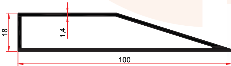
ST 252 0,813 kg/m Alçı Sıva Mastarı GYPSUM PLASTER GAUGE
