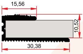
ST 225 0,195 kg/m
