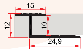
MP 30 0,125 kg/m
