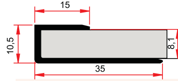
ST 228 0,135 kg/m
