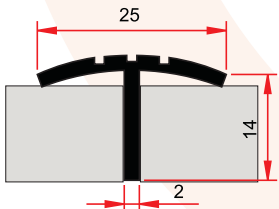
SM 1023 0,188 kg/m
