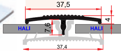
ST 212 0,205 kg/m
