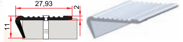
MP 51 0,154 kg/m
