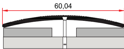
MP 27 0,297 kg/m
