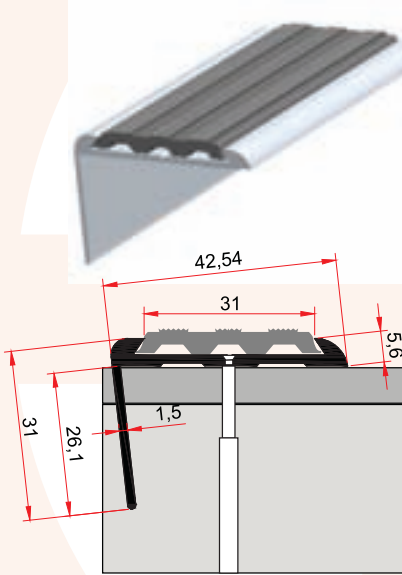
ST 208 0,373 kg/m
