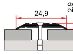
ST 243 0,097 kg/m
