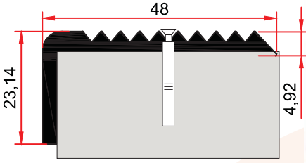
MP 47 0,660 kg/m
