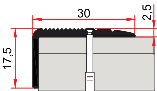
MP 40 0,232 kg/m
