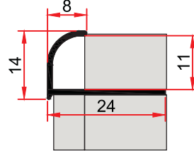
ST 248 D 0,111 kg/m 12 lik Fayans Çıtası 12 MM CERAMIC COVER PROFILE
