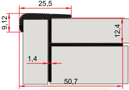
ST 229 B 0,419 kg/m
