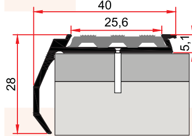
MP 37 0,286 kg/m
