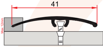
ST 227 A 0,154 kg/m
