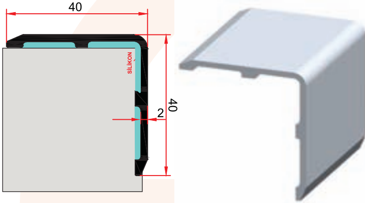
MP 41 0,467 kg/m
