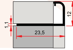
ST 250 A 0,115 kg/m 12 lik Fayans Çıtası 12 MM CERAMIC COVER PROFILE
