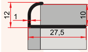
MP 26 0,114 kg/m
