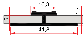
ST 232 A 0,308 kg/m
