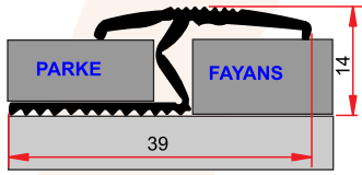
ST 206 0,240 kg/m
