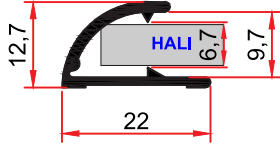
ST 203 0,165 kg/m
