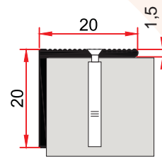
MP 49 0,146 kg/m
