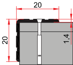
MP 19 0,140 kg/m
