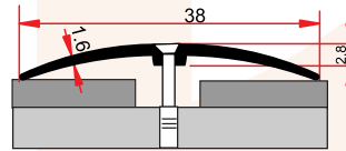
ST 216 0,290 kg/m
