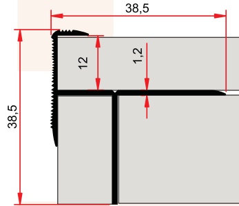
ST 246 B 0,290 kg/m
