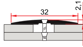
MP 33 0,124 kg/m
