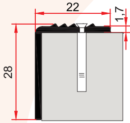
MP 48 0,228 kg/m
