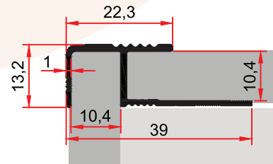
MP 20 0,207 kg/m
