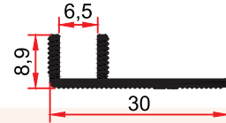
MP 45 0,172 kg/m
