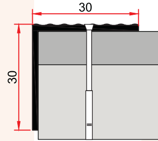
MP 21 0,252 kg/m
