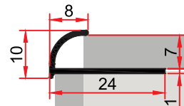
ST 248 B 0,100 kg/m 8 lik Fayans Çıtası 8 MM CERAMIC COVER PROFILE
