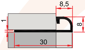
ST 249 0,130 kg/m 6'lik Fayans Çıtası 6 MM CERAMIC COVER PROFILE
