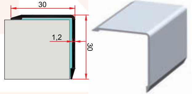
MP 43 0,190 kg/m
