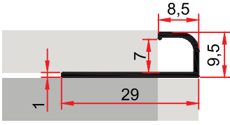
ST 248 0,119 kg/m 8 lik Fayans Çıtası 8 MM CERAMIC COVER PROFILE
