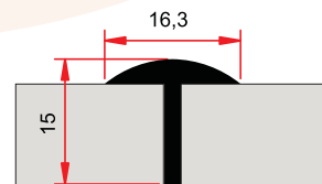
SM 1093 0,145 kg/m
