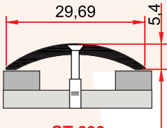
ST 239 0,154 kg/m
