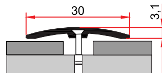
ST 216 B 0,138 kg/m
