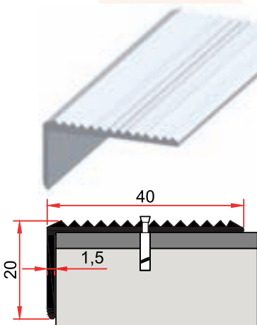
ST 233 0,251 kg/m
