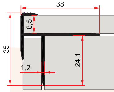
ST 229 0,275 kg/m
