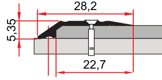
ST 242 0,113 kg/m
