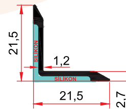
MP 15 0,146 kg/m
