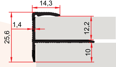
ST 246 D 0,290 kg/m
