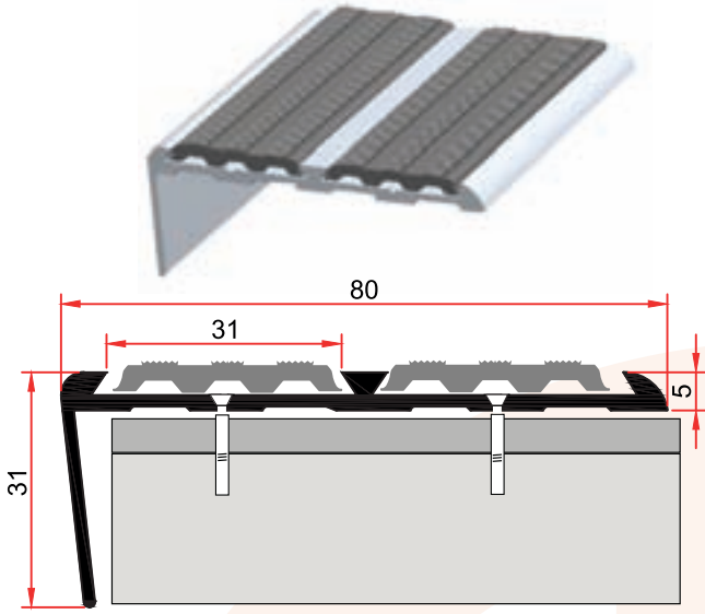
ST 209 0,581 kg/m
