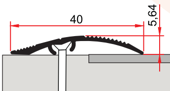
ST 230 C 0,189 kg/m
