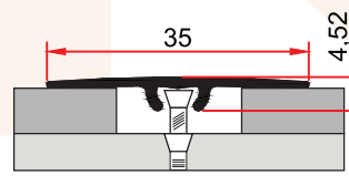
ST 227 B 0,130 kg/m
