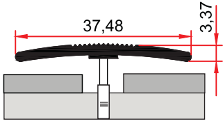
ST 217 0,213 kg/m
