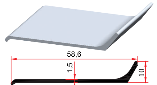
ST 219 L 0,280 kg/m
