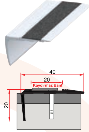
ST 207 A 0,246 kg/m
