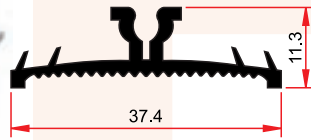
ST 213 (Delikli) 0,350 kg/m Halı Dilatasyon Profili ST 213 DILATATION PROFILE
