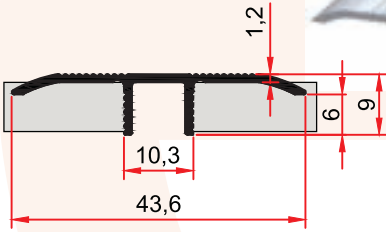
ST 212 E 0,180 kg/m
