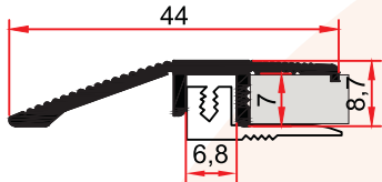
ST 230 0,248 kg/m
