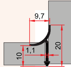
MP 28 0,079 kg/m
