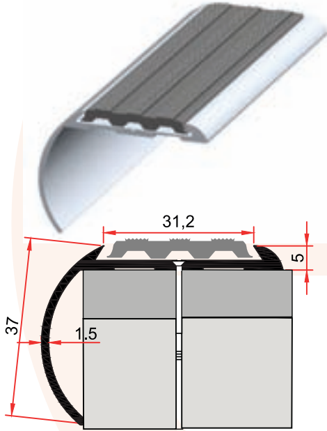
ST 210 0,389 kg/m
