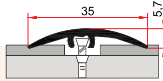
ST 227 0,186 kg/m
