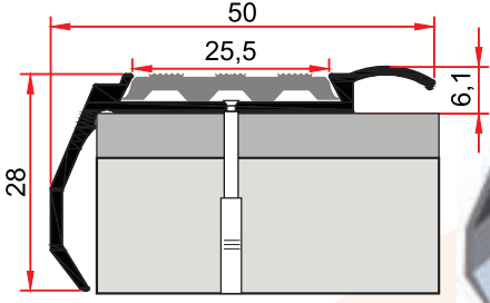
MP 34 0,320 kg/m
