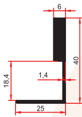
7503 0,485 Kg/m
