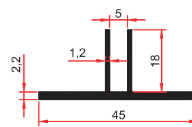
SM 1068 E 0,385 Kg/m
