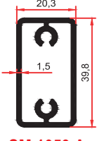
SM 1059 A 0,605 Kg/m
