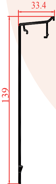
11151 1,045 Kg/m KAPAK PROFİLİ
