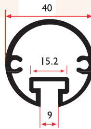
SM 1060 B 0,740 Kg/m
