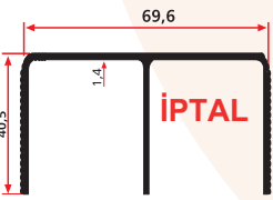
İPTAL SM 1075 B 0,680 Kg/m
