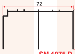
SM 1075 D 0,715 Kg/m
