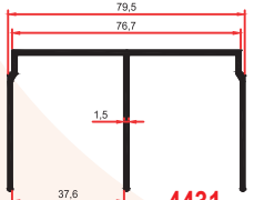
4431 0,825 Kg/m
