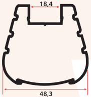
SM 1062 D 0,645 Kg/m
