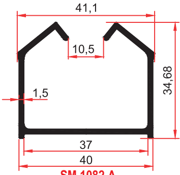
SM 1082 A 0,515 Kg/m
