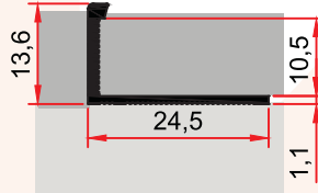
ST 250 E 0,122 kg/m 12 lik Basamak Burunluğu 12 MM STEPNOSE PROFILE
