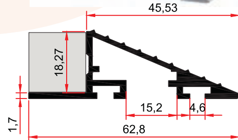
ST 230 R 0,552 kg/m
