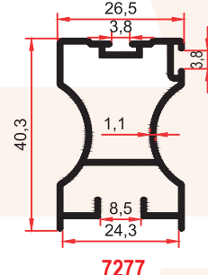
7277 0,480 Kg/m
