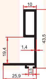
6622 0,405 Kg/m
