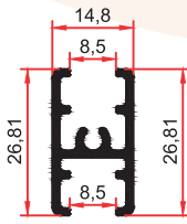
5167 0,320 Kg/m
