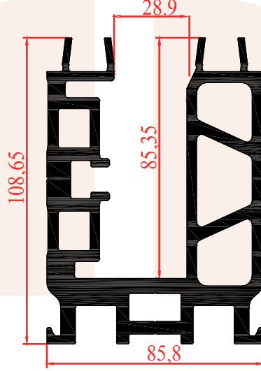
2311 8,155 Kg/m TAŞIYICI PROFİLİ
