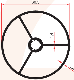
SM 5010 B 1,140 Kg/m
