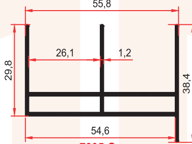
7005 G 0,655 Kg/m
