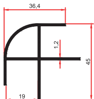
SM 1052 0,485 Kg/m
