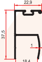
9476 0,295 Kg/m
