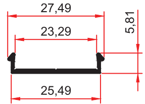
4120 A 0,110 Kg/m
