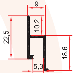
1954 0,145 Kg/m BARİSOL GERGI TAVAN PROFİLİ
