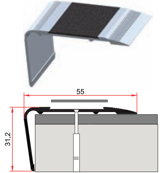
ST 210 A 0,332 kg/m
