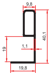
8780 0,275 Kg/m
