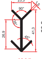
4305 0,370 Kg/m
