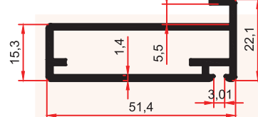
BRN 7358 0,564 Kg/m
