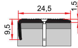
ST 240 A 0,108 kg/m
