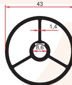
SM 5011 E 0,965 Kg/m
