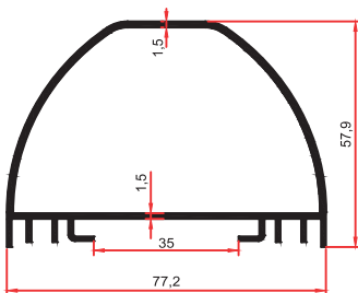
3396 1,065 Kg/m
