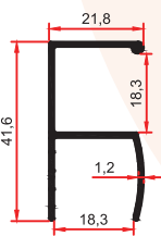
SM 1013 F 0,335 Kg/m
