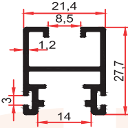
9007 D KULPSUZ 0,375 Kg/m
