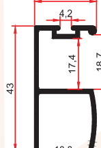
1013 BJ 0,435 Kg/m
