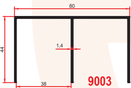
9003 0,740 Kg/m
