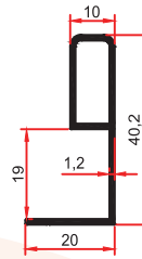
E-1436 0,300 Kg/m
