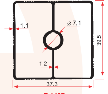
E 1437 0,630 Kg/m
