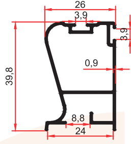
7472 0,375 Kg/m
