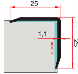
SM 1064 C 0,138 kg/m
