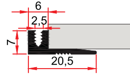
ST 231 0,130 kg/m
