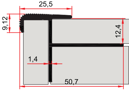
ST 229 B 0,419 kg/m
