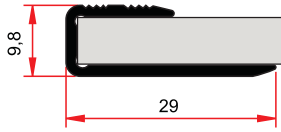
ST 225 B 0,165 kg/m
