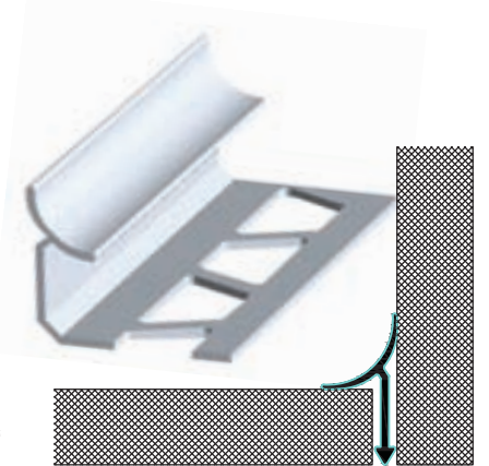
MP 28 0,079 kg/m
