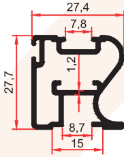
7345 0,470 Kg/m
