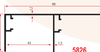
5826 0,785 Kg/m
