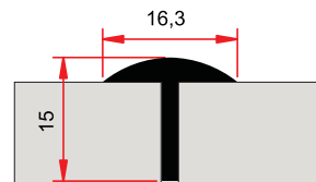
SM 1093 0,145 kg/m
