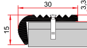
MP 50 0,316 kg/m
