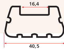
SM 1062 K 0,425 Kg/m
