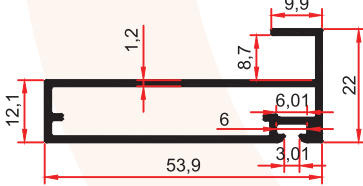
7575 0,524 Kg/m
