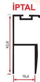
E 1066 0,405 Kg/m
