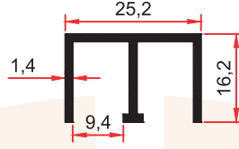
2109 0,275 Kg/m
