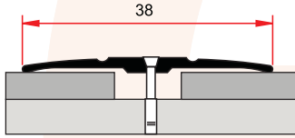
MP 6 0,137 kg/m
