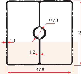
E 1438 0,775 Kg/m
