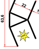
SM 1052 J 0,565 Kg/m
