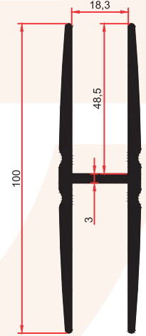
SM 1062 H 1,895 Kg/m
