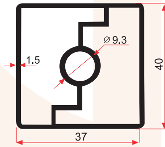
E 1042 0,955 Kg/m
