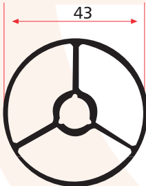
SM 5014 B 0,820 Kg/m
