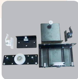
SGM 02 Dış Kanat Rulmanı SGM 02 İç Kanat Rulmanı
