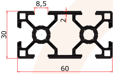
FS 4013 D 1,410 Kg/m
