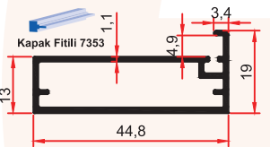
7353 0,421 Kg/m
