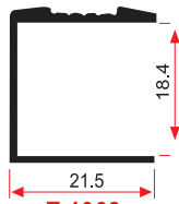
E 1968 0,205 Kg/m
