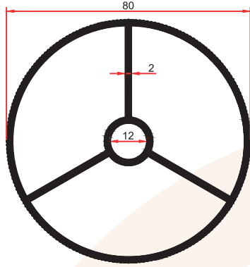
SM 5010 A 1,990 Kg/m
