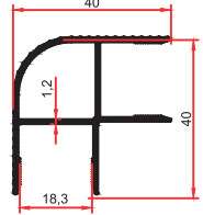
SM 1052 E 0,551 Kg/m
