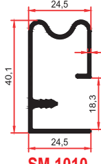
SM 1010 0,455 Kg/m
