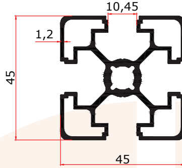
FS 4013 B 1,235 Kg/m
