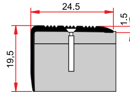
ST 241 A 0,138 kg/m
