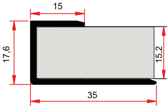
ST 228 A 0,215 kg/m
