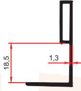
8800 0,305 Kg/m
