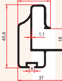
SM 1013 BE 0,515 Kg/m
