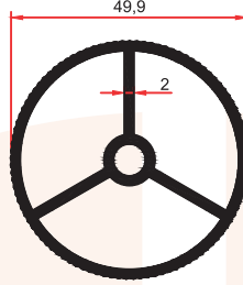
SM 5010 1,215 Kg/m
