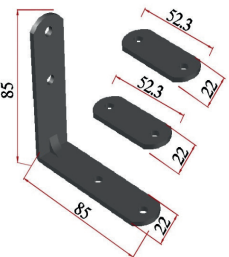
4479 SAC KÖŞE
