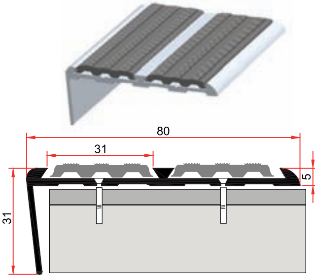
ST 209 0,581 kg/m
