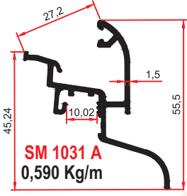
SM 1031 A Damlalık Tapası
