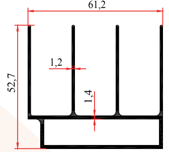
SSC-1003 1,050 Kg/m SÜRME ÜST RAY
