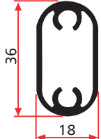
SM 1059 C 0,510 Kg/m
