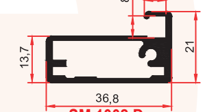
SM 1002 D 0,550 Kg/m
