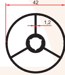
SM 5014 D 0,760 Kg/m
