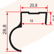
SM 1011 B 0,215 Kg/m
