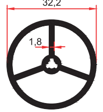
E 1049 0,690 Kg/m
