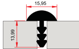
SM 1023 B 0,180 kg/m
