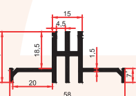
1068 Ç 0,640 Kg/m
