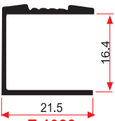
E 1988 0,205 Kg/m
