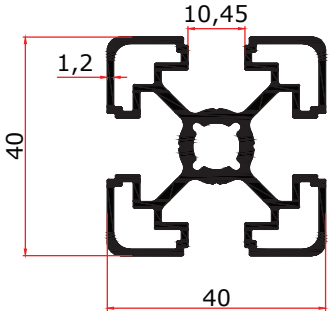
FS 4013 A 1,090 Kg/m
