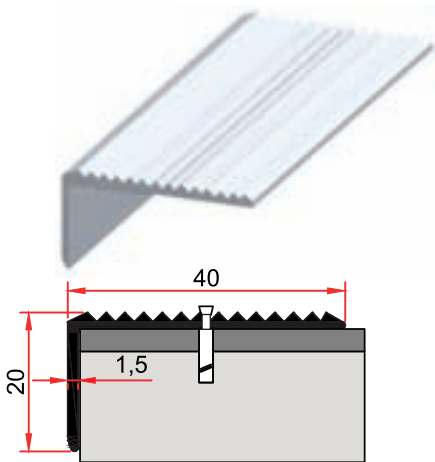
ST 233 0,251 kg/m
