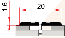
MP 1 0,085 kg/m
