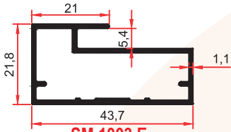
SM 1003 E 0,462 Kg/m
