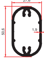
SM 1059 B 0,860 Kg/m
