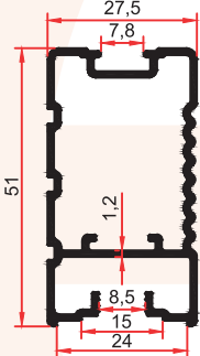
7349 0,655 Kg/m
