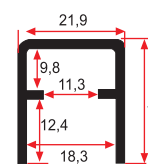
SM 1012 A 0,350 Kg/m
