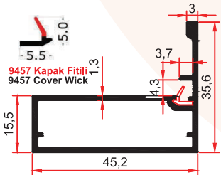
8976 0,529 Kg/m
