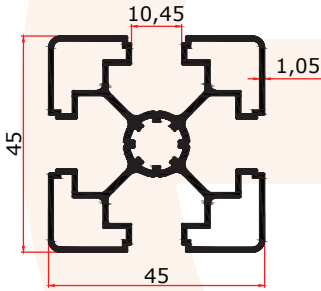
FS 4013 F 1,025 Kg/m
