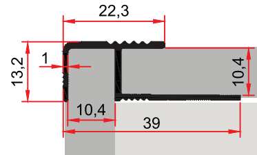
MP 20 0,207 kg/m
