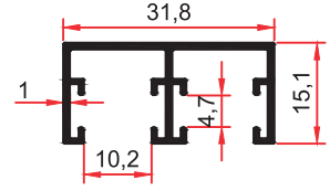
2109 A 0,265 Kg/m
