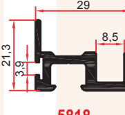
5818 0,430 Kg/m
