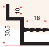
SM 1038 SA 0,485 Kg/m
