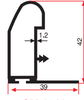
SM 1011 0,490 Kg/m
