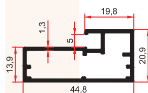
7630 0,512 Kg/m
