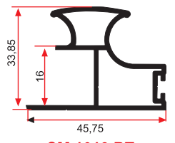
SM 1013 BT 0,280 Kg/m
