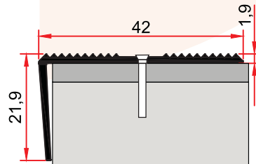
ST 244 0,231 kg/m
