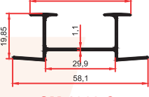
SM 1068 C 0,325 Kg/m
