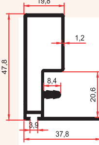
BRN 7356 0,605 Kg/m
