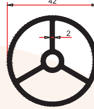
SM 5011 1,020 Kg/m
