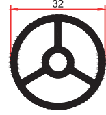
SM 5012 0,775 Kg/m
