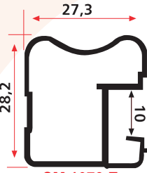
SM 1073 E 0,365 Kg/m
