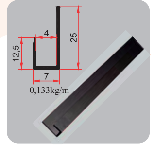
S-LCW U Çıta boy 300cm
