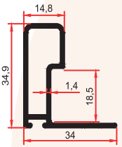
SM 1013 BA 0,445 Kg/m
