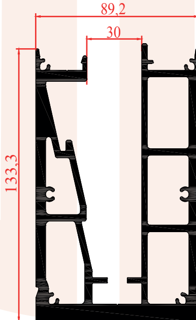
11153 9,265 Kg/m TAŞIYICI PROFİLİ
