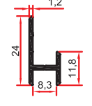
4460 0,145 Kg/m
