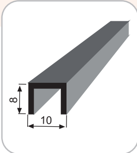
Süpürgelik U Fugası
