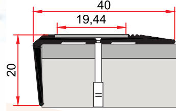
MP 35 0,246 kg/m
