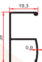
3796 A 0,235 Kg/m
