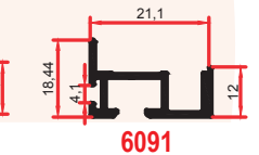
6091 0,290 Kg/m
