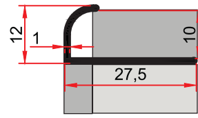
MP 26 0,114 kg/m
