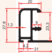
SM 1012 B 0,425 Kg/m
