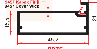
8975 0,458 Kg/m
