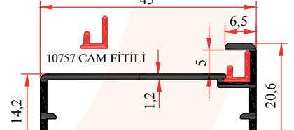
10757 0,470 Kg/m
