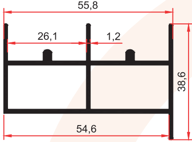
7005 H 0,735 Kg/m
