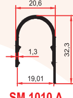
SM 1010 A 0,230 Kg/m
