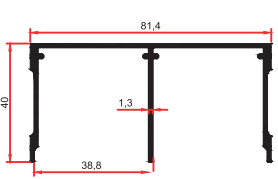
SM 1075 A 0,805 Kg/m
