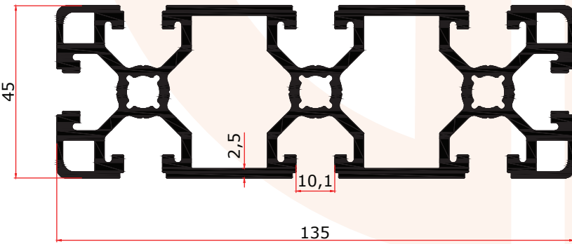
FS 4013 N 4,535 Kg/m
