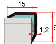
MP 32 0,092 kg/m
