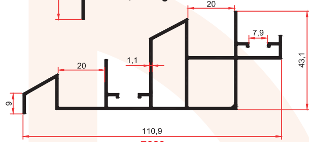
7689 1,005 Kg/m
