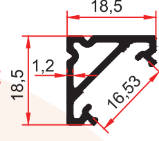
3729 A 0,230 Kg/m
