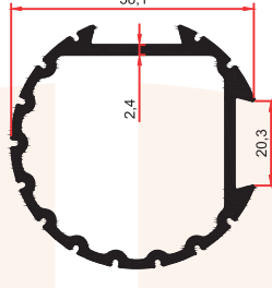
SM 1062 B 1,305 Kg/m
