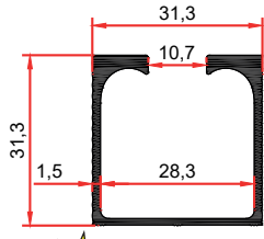
6684 0,498 Kg/m
