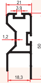
SM 1013 BK 0,495 Kg/m
