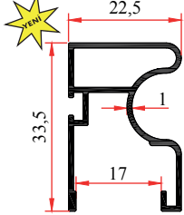
5882 A 0,335 Kg/m
