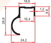
SM 1011 K 0,215 Kg/m
