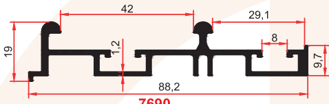
7690 0,786 kg/m
