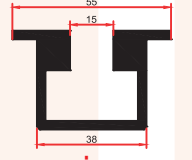
ARÇELİK KANALI 1,605 Kg/m
