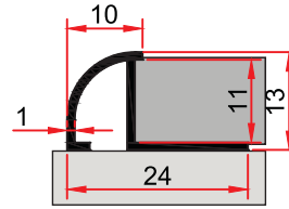
ST 248 F 0,130 kg/m
