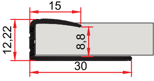
ST 214 0,168 kg/m
