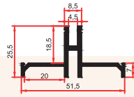
1068 H 0,495 Kg/m
