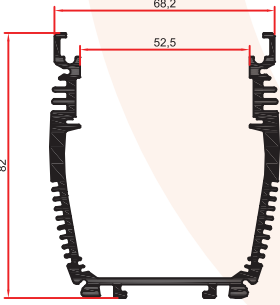
4664 2,030 Kg/m
