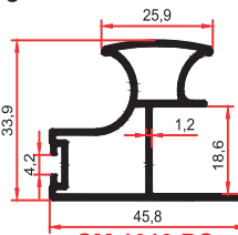
SM 1013 BS 0,585 Kg/m
