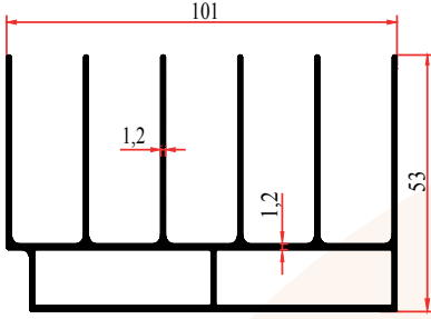
SSC-1000 1,550 Kg/m SÜRME ÜST RAY
