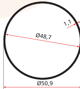
SM 5014 E 0,465 Kg/m
