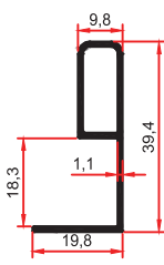
SM 1010 P 0,275 Kg/m
