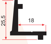
SM 1084 0,345 Kg/m
