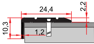
ST 240 0,151 kg/m
