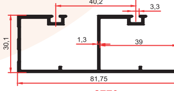
8770 0,870 Kg/m
