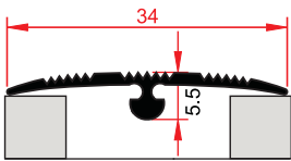
ST 212 B 0,164 kg/m
