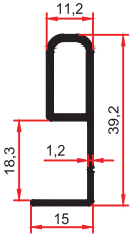
6065 0,325 Kg/m
