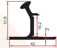
SM 1013 M 0,545 Kg/m
