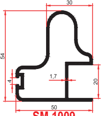
SM 1009 0,945 Kg/m
