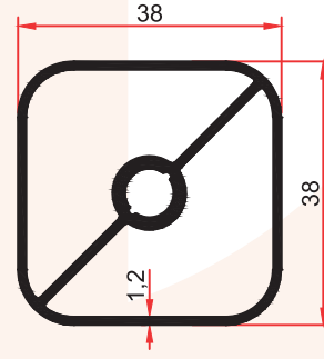
6289 0,680 Kg/m
