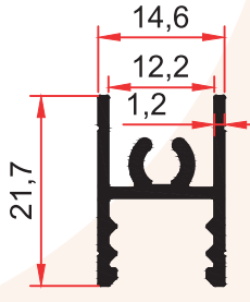
SM 1076 E 0,250 Kg/m
