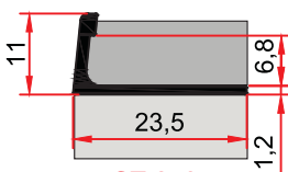
ST 250 0,124 kg/m Basamak Burunluğu STEPNOSE PROFILE
