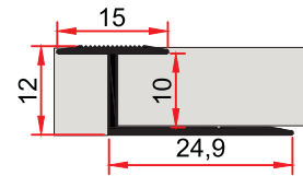
MP 30 0,125 kg/m
