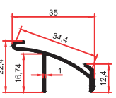
SM 1030 0,215 Kg/m
