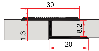
ST 245 0,186 kg/m
