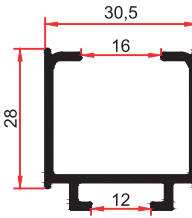
SM 1092 B 0,445 Kg/m
