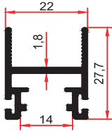
9007 A 0,395 Kg/m
