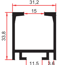
SM 1092 0,567 Kg/m
