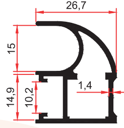
SM 1073 A 0,470 Kg/m
