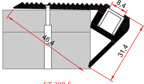
ST 208 S 0,683 kg/m
