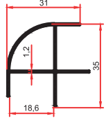
SM 1052 F 0,385 Kg/m
