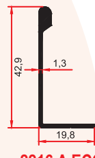
2216 A ECO 0,275 Kg/m
