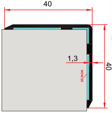
SM 1064 A 0,302 kg/m
