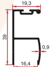
3797 A 0,255 Kg/m
