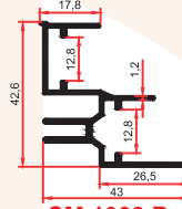
SM 1088 B 0,555 Kg/m
