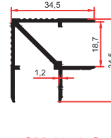
SM 1052 G 0,400 Kg/m
