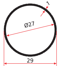
SM 5014 F 0,235 Kg/m
