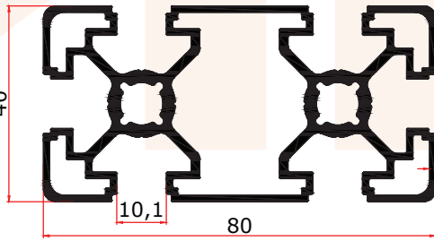
FS 4013 E 1,955 Kg/m
