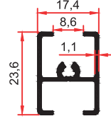
8062 0,255 Kg/m
