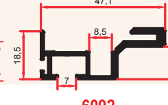
6092 0,485 Kg/m
