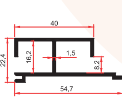
SM 1044 C 0,545 Kg/m
