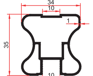
SM 1073 B 0,500 Kg/m
