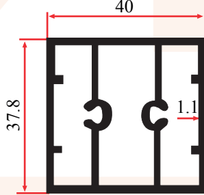
SK 707 0,760 Kg/m
