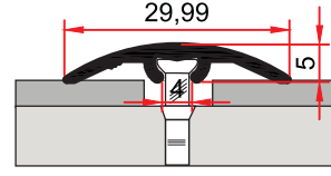
MP 5 0,140 kg/m
