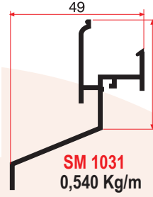
SM 1031 A Damlalık Fitili
