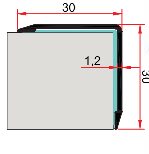
MP 43 0,190 kg/m
