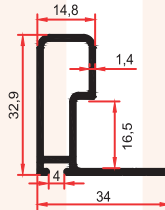
SM 1013 BC 0,435 Kg/m
