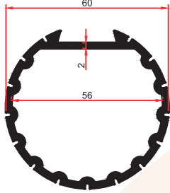
SM 1062 1,205 Kg/m
