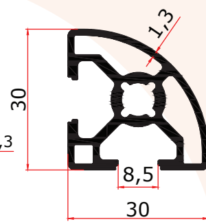
FS 4013 G 0,675 Kg/m
