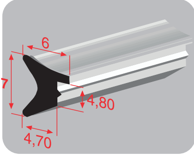
Cam Fitili Orta (Şeffaf)
