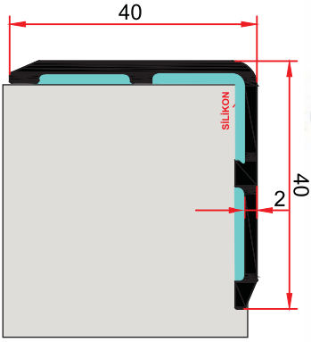
MP 41 0,467 kg/m
