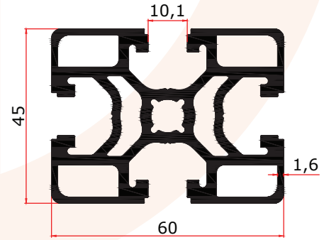
FS 4013 P 2,525 Kg/m
