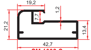
SM 1002 C 0,445 Kg/m
