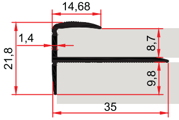
ST 246 E 0,227 kg/m
