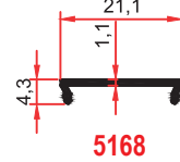
5168 0,115 Kg/m
