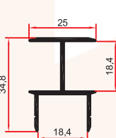
2444 0,565 Kg/m
