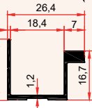
1936 0,240 Kg/m
