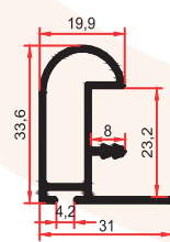
SM 1012 E 0,455 Kg/m
