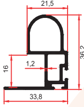
SM 1013 D 0,475 Kg/m
