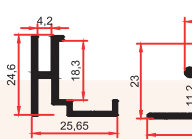
1068 G 0,335 Kg/m
