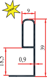
1010 P EKO 0,215 Kg/m
