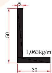
S-WKK Ayna çerçevesi boy:600cm
