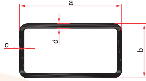
RADİUSLU DİKDÖRTGEN BORULAR
