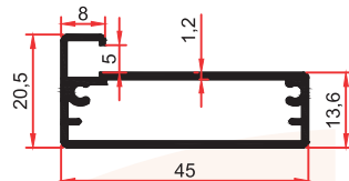
SM 1002 A 0,456 Kg/m
