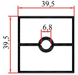
SK 703 0,795 Kg/m
