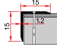
ST 234 B 0,090 kg/m
