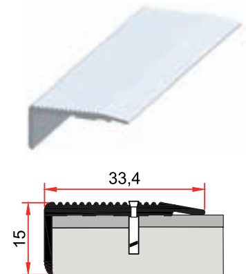
ST 233 A 0,230 kg/m
