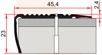
MP 38 0,284 kg/m
