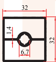
SK 710 0,630 Kg/m
