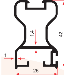
5804 0,495 Kg/m
