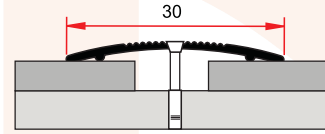
MP 31 0,090 kg/m
