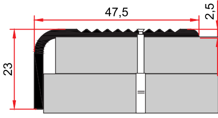
MP 46 0,398 kg/m
