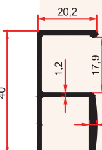
SM 1013 BF 0,365 Kg/m
