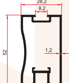
13436 0,625 Kg/m
