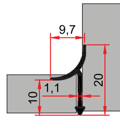
MP 28 0,079 kg/m
