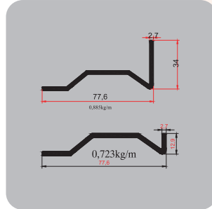
S-LCW Duvar dikme boy 274 cm
