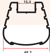
SM 1062 F 0,645 Kg/m
