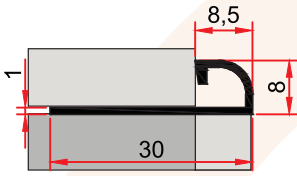
ST 249 0,130 kg/m 6'lık Fayans Çıtası 6 MM CERAMIC COVER PROFILE
