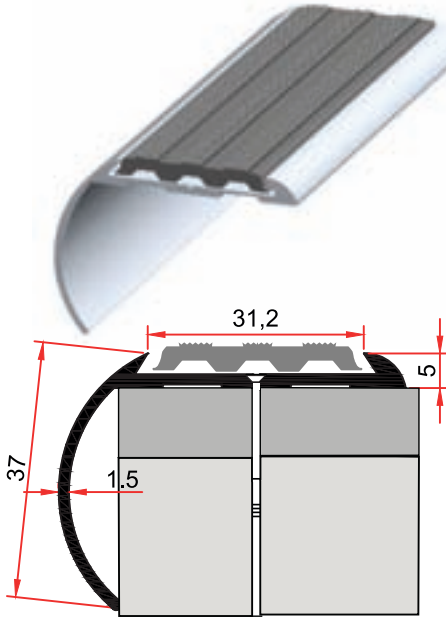
ST 210 0,389 kg/m
