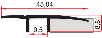
MP 44 0,199 kg/m
