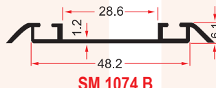
SM 1074 B 0,325 Kg/m
