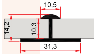
ST 232 0,227 kg/m
