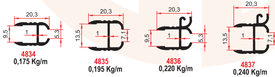
Yazı tahta köşesi 8'lik
