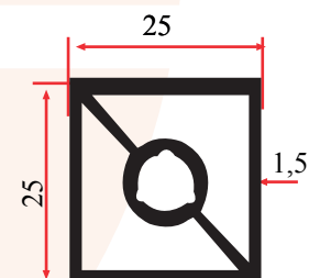
SK 706 0,585 Kg/m
