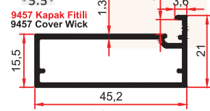
9457 0,453 Kg/m
