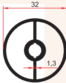
SM 5014 C 0,550 Kg/m
