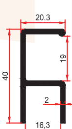
SM 1013 A 0,505 Kg/m
