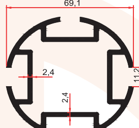
SB 5016 2,235 Kg/m
