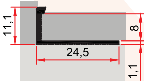
ST 250 D 0,111 kg/m 10 luk Basamak Burunluğu 10 MM STEPNOSE PROFILE
