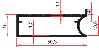
7352 B 0,485 Kg/m
