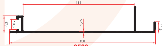
9583 0,985 Kg/m
