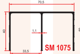
SM 1075 0,575 Kg/m
