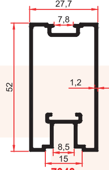
7348 0,645 Kg/m
