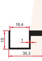
8965 0,255 Kg/m
