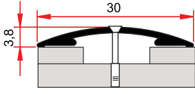
ST 239 B 0,130 kg/m
