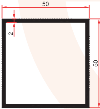
SK 712 0 988 kg/m
