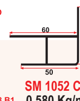
SM 1052 C 0,580 Kg/m
