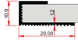
ST 225 A 0,144 kg/m
