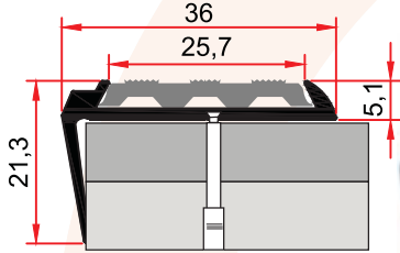
MP 36 0,246 kg/m
