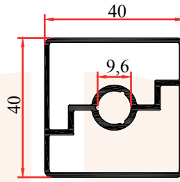
SK 701 0,855 Kg/m
