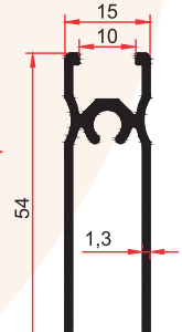
SM 1072 B 0,490 Kg/m
