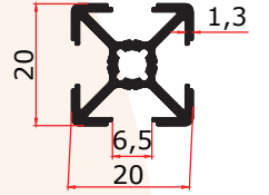
FS 4013 H 0,345 Kg/m
