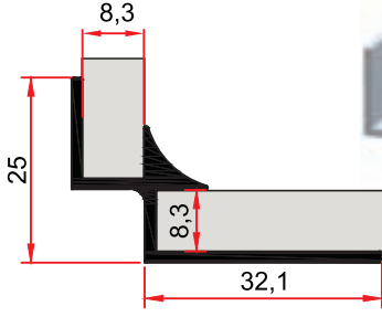
ST 229 A 0,340 kg/m
