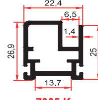
7005 K 0,475 Kg/m
