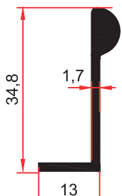
SM 1082 B 0,300 Kg/m
