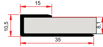
ST 228 0,135 kg/m
