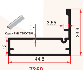
7350 0,497 Kg/m
