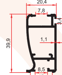
7347 0,430 Kg/m
