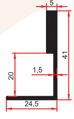
9126 A 0,445 Kg/m
