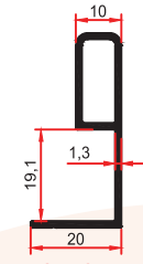
8756 0,325 Kg/m
