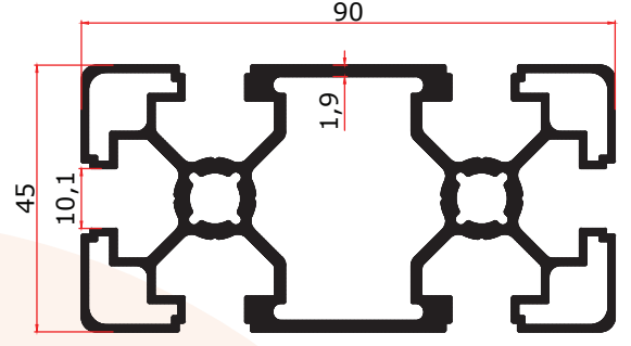
FS 4013 C 2,330 Kg/m
