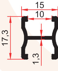
SM 1071 D 0,180 Kg/m
