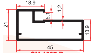
SM 1007 B 0,450 Kg/m
