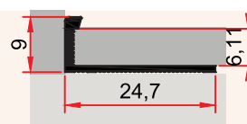
ST 250 B 0,103 kg/m 8 lik Basamak Burunluğu 8 MM STEPNOSE PROFILE
