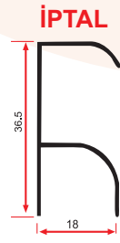
E 1910 0,225 Kg/m
