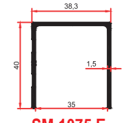
SM 1075 E 0,490 Kg/m
