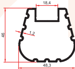
SM 1062 C 0,635 Kg/m
