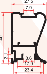
13431 0,515 Kg/m
