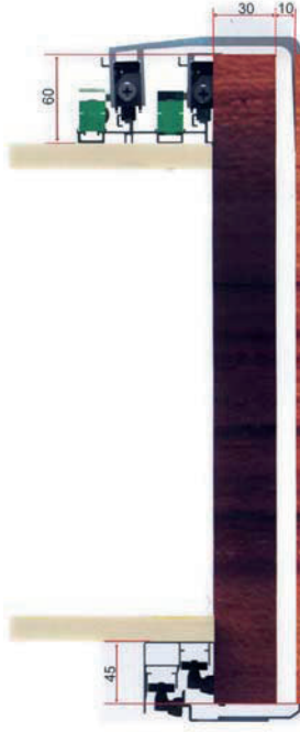
Ayarlı Dış Üst Makara
