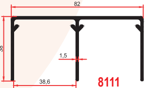
8111 0,845 Kg/m
