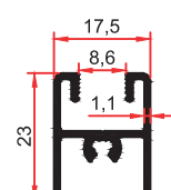
6830 0,265 Kg/m
