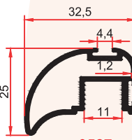
9527 0,385 Kg/m
