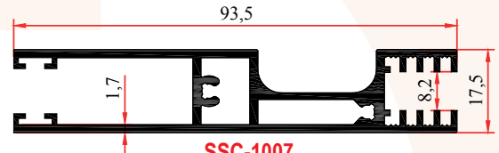
SSC-1007 1,250 Kg/m SÜRME ALT ETEK-8MM
