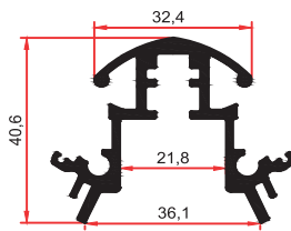
5293 0,950 Kg/m
