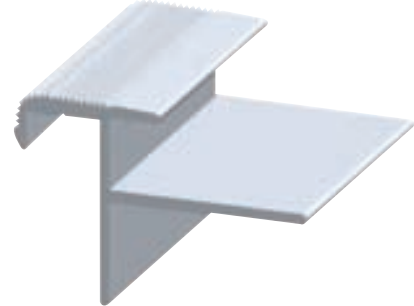
ST 246 D 0,290 kg/m
