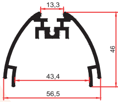
SM 1067 G 0,825 Kg/m
