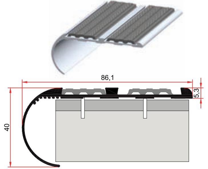
ST 211 0,709 kg/m
