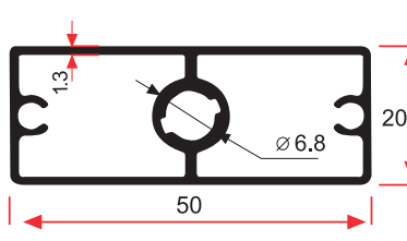
E 1001 0,700 Kg/m
