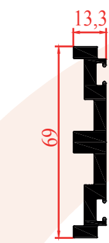
2312 1,370 Kg/m SIKIŞTIRMA PROFİLİ
