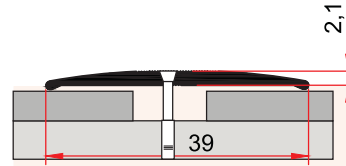
MP 7 0,172 kg/m
