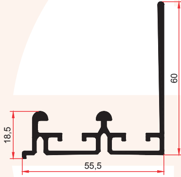
11813 A 0,885 Kg/m
