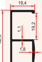
6066 0,305 Kg/m
