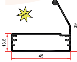
PRF-30075 0,505 Kg/m
