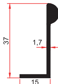
SM 1082 C 0,320 Kg/m
