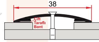
ST 239 C 0,132 kg/m
