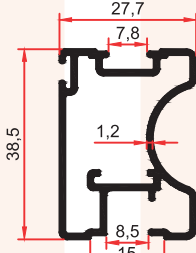
7346 0,565 Kg/m
