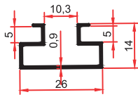
8585 0,175 Kg/m
