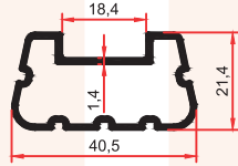
SM 1062 G 0,450 Kg/m
