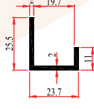
SM 1055 D 0,310 Kg/m
