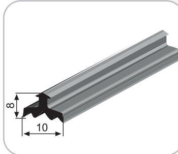
3002 Fitil Baskı Çıtası
