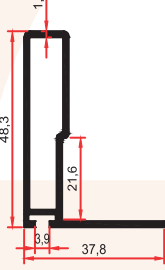
12839 0,565 Kg/m
