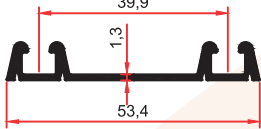
6010 A 0,355 Kg/m
