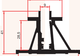
6457 1,445 Kg/m
