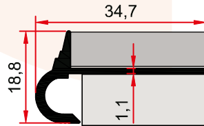
ST 253 C 0,216 kg/m Süslü Basamak Burunluđu STEPMOSE PROFILE
