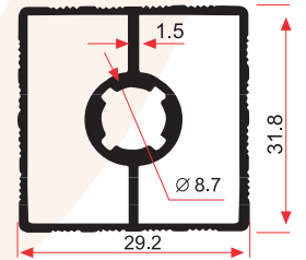
E 1008 0,675 Kg/m
