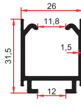
SM 1092 A 0,424 Kg/m
