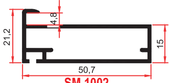
SM 1002 0,495 Kg/m
