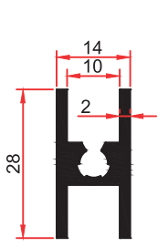
SM 1071 A 0,435 Kg/m
