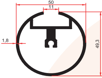
SM 5014 1,100 Kg/m Yönlendirme Dikmesi
