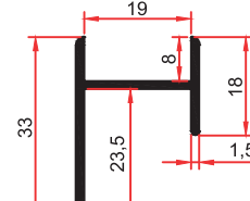
SM 1027 B 0,275 Kg/m
