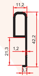
SM 1010 B 0,295 Kg/m
