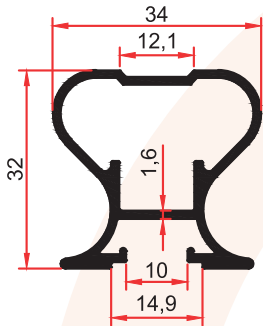
SM 1073 D 0,525 Kg/m
