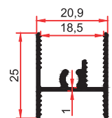
7475 0,245 Kg/m
