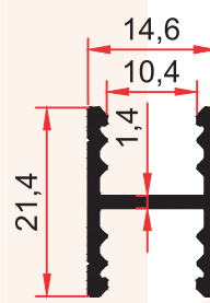
SM 1071 E 0,220 Kg/m
