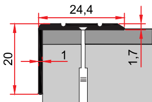
ST 241 0,151 kg/m
