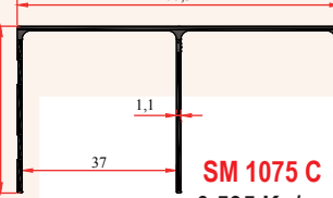
SM 1075 C 0,595 Kg/m
