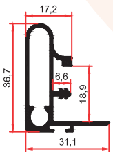
SM 1012 C 0,455 Kg/m
