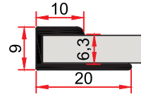
ST 215 0,124 kg/m
