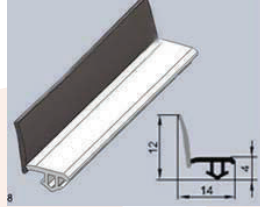
SM 1031 A Damlalık Fitili
