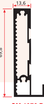
SM 1076 D 1,030 Kg/m
