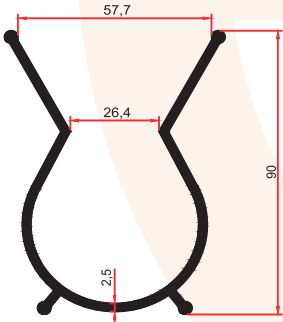
SM 1061 M 1,620 Kg/m
