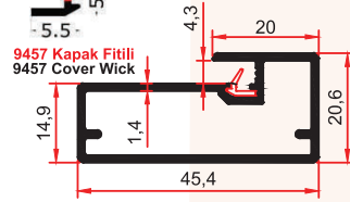
SM 1007 P 0,548 Kg/m
