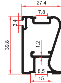
7344 0,550 Kg/m
