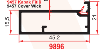
9896 0,465 Kg/m
