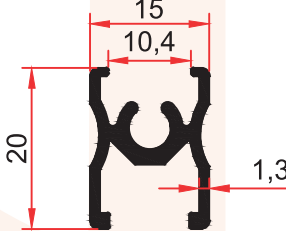
SM 1076 K 0,255 Kg/m
