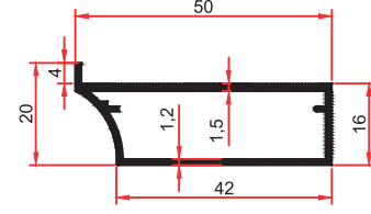
7352 C 0,445 Kg/m
