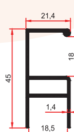
SM 1013 0,485 Kg/m
