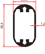
SM 1059 D 0,660 Kg/m
