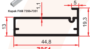
7351 0,421 Kg/m
