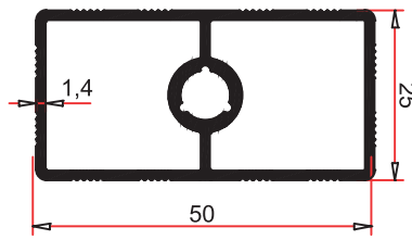
6514 0,695 Kg/m
