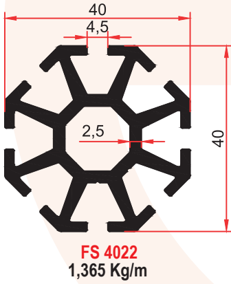
40x40 Sigma Bağlantı
