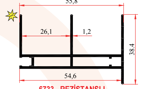
6733 - REZİSTANSLI 0,670 Kg/m
