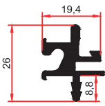
SM 1038 B 0,415 Kg/m
