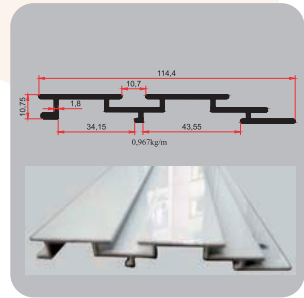
S-LCW Lambiri boy 600cm 12717 - 0,967gr/m
