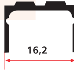
SM 1062 Ç2 0,135 Kg/m
