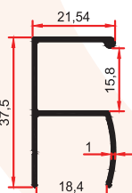
9475 0,265 Kg/m
