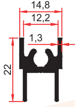
SM 1076 A 0,290 Kg/m
