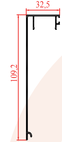
2313 0,630 Kg/m KAPAK PROFİLİ
