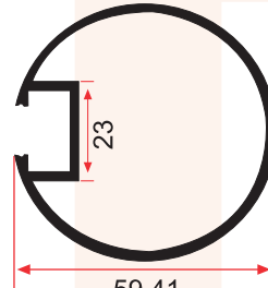
SM 1060 0,155 Kg/m
