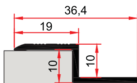
SM 1064 B 0,193 kg/m
