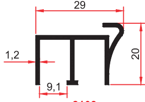
2108 0,290 Kg/m
