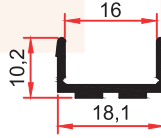
SM 1062 Ç1 0,135 Kg/m
