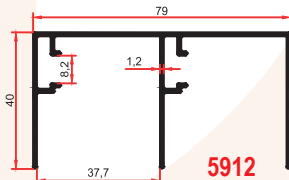
5912 0,735 Kg/m
