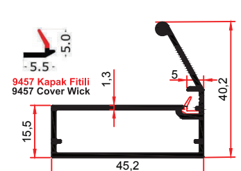
3638 A 0,556 Kg/m
