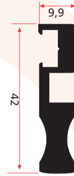
SM 1076 F 0,710 Kg/m
