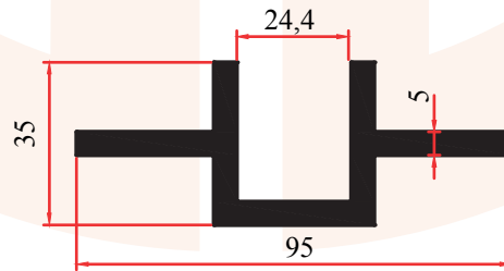
SB 5039 2,095 Kg/m Özel Kutu Orta Bağlantı
