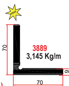
Kapı Kasası Dışlı Köşe
