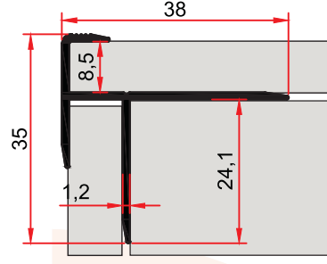
ST 229 0,275 kg/m
