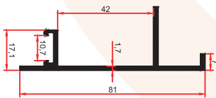
SM 1027 E 0,645 Kg/m
