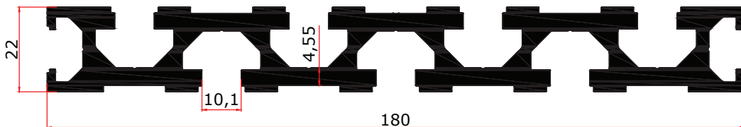
FS 4013 R 5,055 Kg/m
