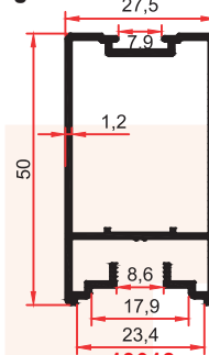
13018 0,570 Kg/m
