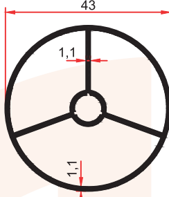
E 1097 0,715 Kg/m
