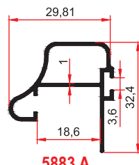
5883 A 0,305 Kg/m
