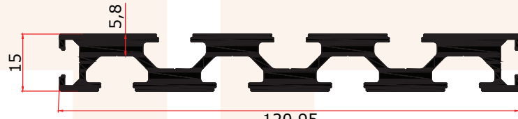
FS 4013 M 2,320 Kg/m
