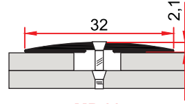
MP 33 0,124 kg/m
