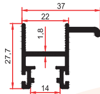
9007 B 0,485 Kg/m
