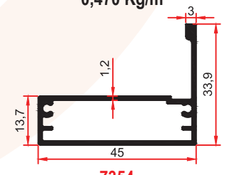
7354 0,505 Kg/m
