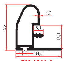
SM 1011 A 0,480 Kg/m
