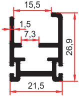
7005 F 0,400 Kg/m
