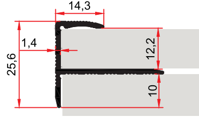
ST 246 D 0,290 kg/m
