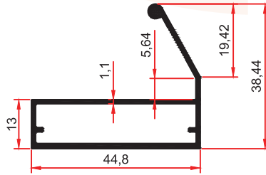
8599 0,491 Kg/m
