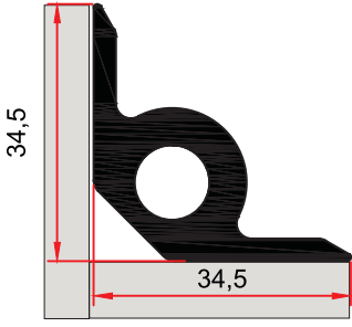
SM 2011 0,926 kg/m
