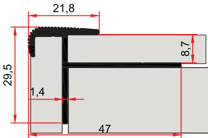
ST 229 D 0,381 kg/m
