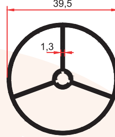
E 1163 0,715 Kg/m
