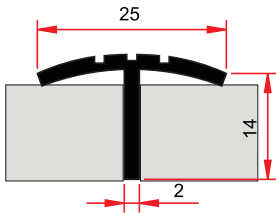
SM 1023 0,188 kg/m
