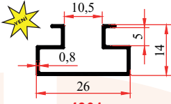
4301 0,160 Kg/m
