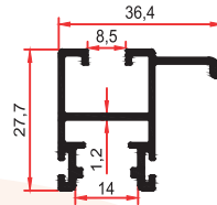
9007 E KULPLU 0,440 Kg/m
