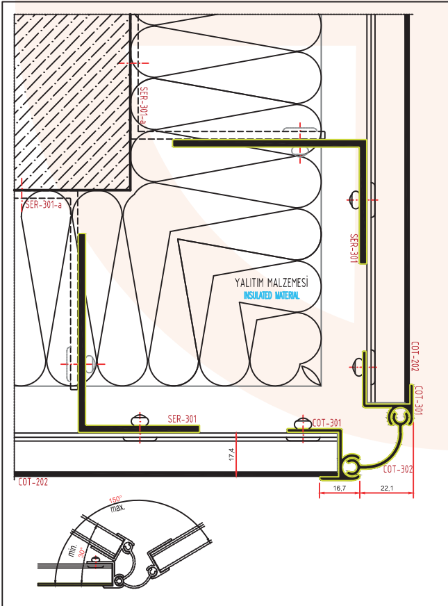
KÖŞE DETAY CORNER DETAIL
