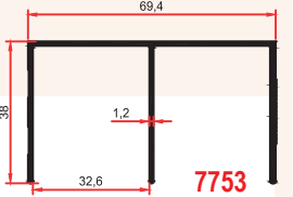
7753 0,625 Kg/m
