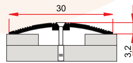
ST 239 G 0,103 kg/m
