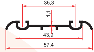
SM 1074 E 0,245 Kg/m
