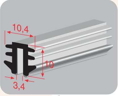
U Cam Fitili İnce (Şeffaf)
