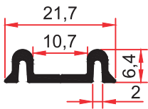
7307 0,140 Kg/m
