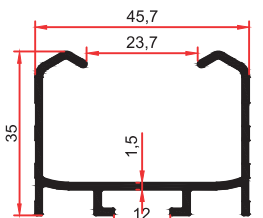
SM 1092 C 0,566 Kg/m
