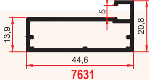
7631 0,460 Kg/m
