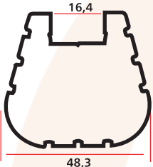
SM 1062 E 0,645 Kg/m
