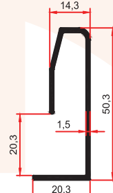
SM 1013 Y 0,425 Kg/m
