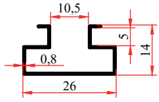
4301 0,160 Kg/m
