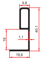
8780 0,275 Kg/m
