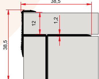
ST 246 B 0,290 kg/m
