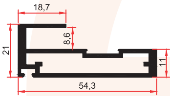
SM 1002 E 0,720 Kg/m
