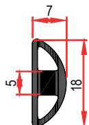
PRF-30326 0,180 Kg/m
