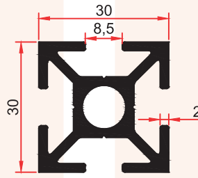
FS 4016 A 0,925 Kg/m
