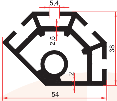
FS 4023 1,505 Kg/m
