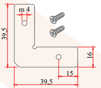
Köşe Birleştirme Aparatı
