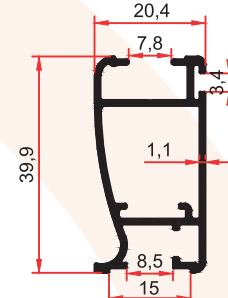
7347 0,430 Kg/m
