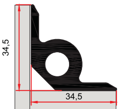
SM 2011 0,926 kg/m
