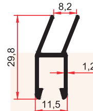
2110 B 0,240 Kg/m
