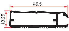
SM 1000 A 0,395 Kg/m
