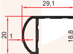
4746 0,185 Kg/m
