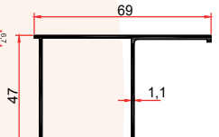
4530 0,630 Kg/m
