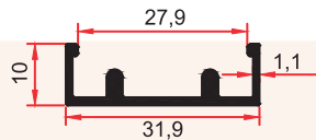
2112 A 0,235 Kg/m
