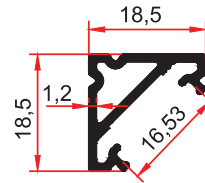
3729 A 0,230 Kg/m
