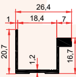
1936 0,240 Kg/m
