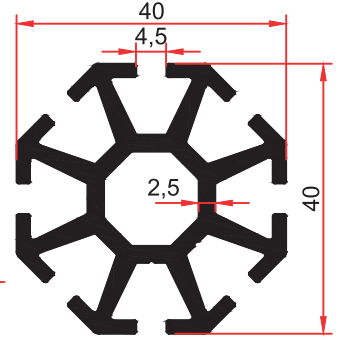
FS 4022 1,365 Kg/m
