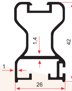
5804 0,495 Kg/m
