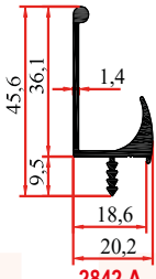
2842 A 0,385 Kg/m
