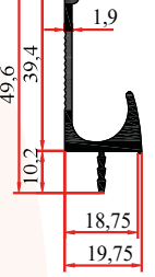
1012 ÇD 0,495 Kg/m
