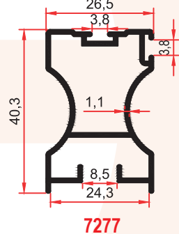
7277 0,480 Kg/m
