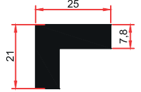
E 1068 0,805 Kg/m
