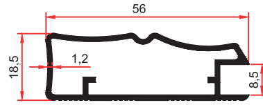
SM 1000 C 0,545 Kg/m
