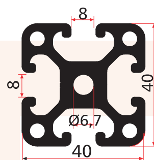
FS 4012 B 2,065 Kg/m
