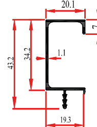
PRF-30446 0,280 Kg/m
