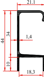
SM 1013 G2 0,390 Kg/m
