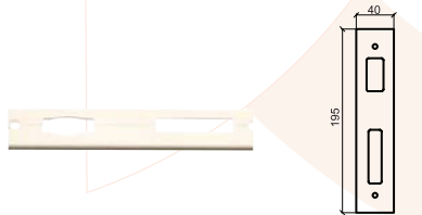
Aldoks Dilli Kilit Karşılığı Locking Plate
