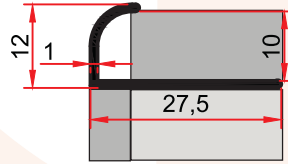
MP 26 0,114 kg/m
