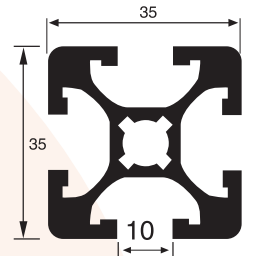
FS 4015 1,340 Kg/m
