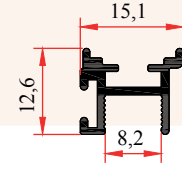
SSC-1009 0,150 Kg/m SÜRME ÜST ETEK-8MM
