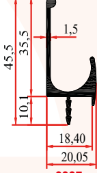
8227 0,420 Kg/m
