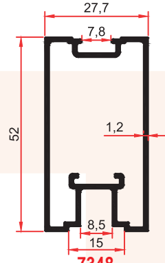
7348 0,645 Kg/m
