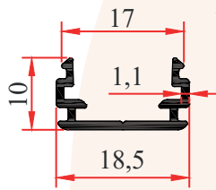
PRF-30400 0,130 Kg/m
