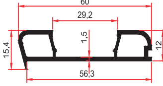
SM 1014 T6 0,485 Kg/m
