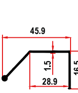
7327 BRN 0,325 Kg/m
