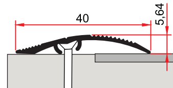
ST 230 C 0,189 kg/m
