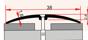
ST 216 0,290 kg/m
