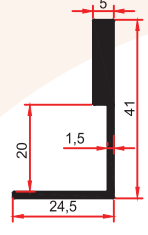
9126 A 0,445 Kg/m
