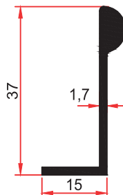
SM 1082 C 0,320 Kg/m
