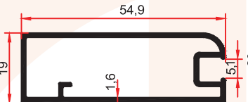
7355 0,575 Kg/m
