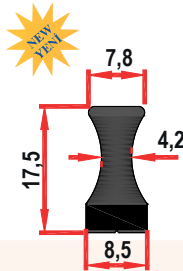
PRF-30327 0,300 Kg/m
