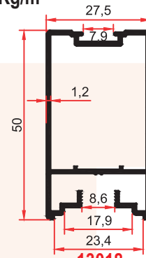
13018 0,570 Kg/m
