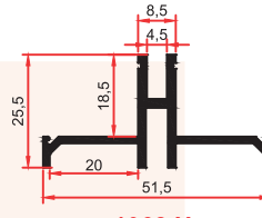
1068 H 0,495 Kg/m
