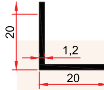
ST 235 0,124 kg/m
