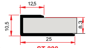
ST 228 0,135 kg/m
