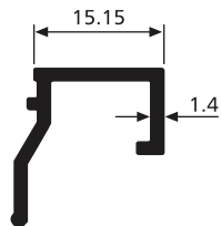
SD 1412 0,170 Kg/m
