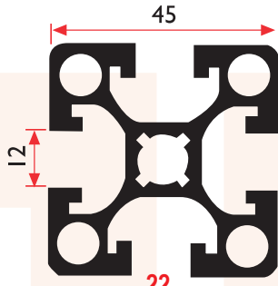
FS 4012 B 2,065 Kg/m
