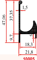
10005 0,535 Kg/m
