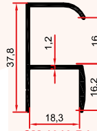
SM 1013 B1 0,320 Kg/m
