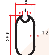
SM 1063M 0,255kg/m
