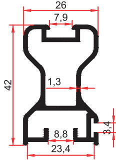
4418 0,600 Kg/m
