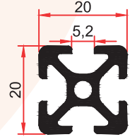
FS 4018 0,465 Kg/m
