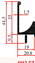
1013 ÇZ 0,520 Kg/m
