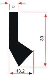
E 1945 0,495 Kg/m
