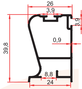
7472 0,375 Kg/m
