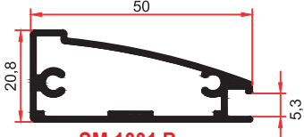
SM 1001 B 0,570 Kg/m
