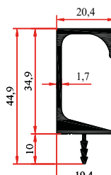
SM 1013 G EKO-1 0,540 Kg/m
