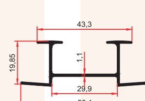
SM 1068 C 0,325 Kg/m
