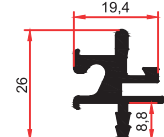
SM 1038 B 0,415 Kg/m
