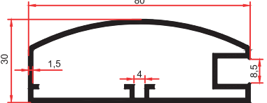
SM 1001 C 0,955 Kg/m
