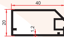
SM 1013 EK 0,435 Kg/m
