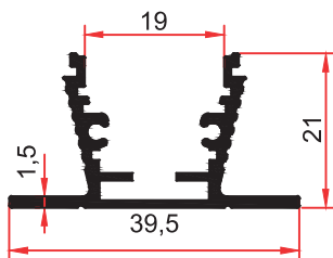
3735 0,375 Kg/m
