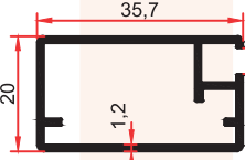
SM 1003 DK 0,395 Kg/m
