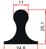
SM 6013 G 0,695 Kg/m
