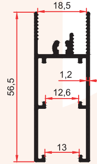
7474 0,530 Kg/m
