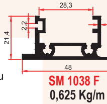
Işıklı raf (ölçüye göre imalat yapılır)
