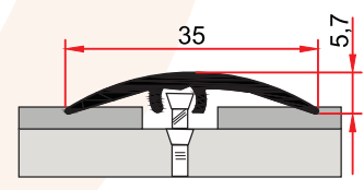
ST 227 0,186 kg/m
