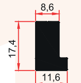
SM 6014 CR 0,445 Kg/m
