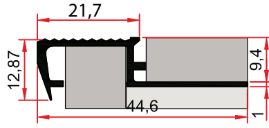
ST 253 0,257 kg/m Basamak Burunluğu STEPMOSE PROFILE
