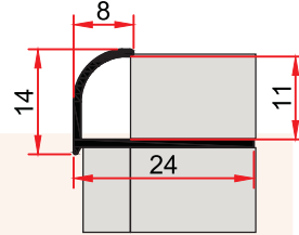
ST 248 D 0,111 kg/m 12 lik Fayans Çıtası 12 MM CERAMIC COVER PROFILE
