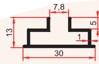
SM 1041 0,190 Kg/m
