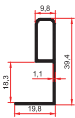
SM 1010 P 0,275 Kg/m
