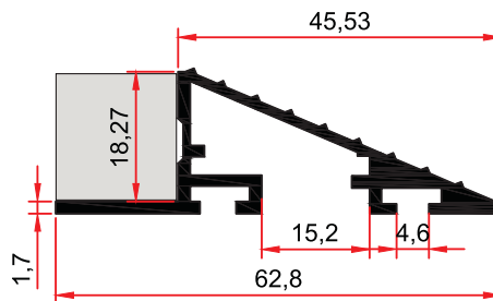
ST 230 R 0,552 kg/m
