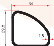
SB 5030 A 0,500 Kg/m
