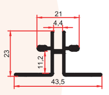
1068 B 0,410 Kg/m
