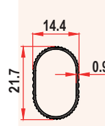
12050 0,120 Kg/m
