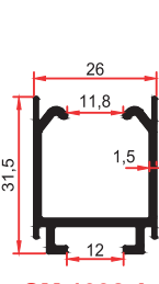
SM 1092 A 0,424 Kg/m
