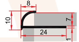
ST 248 B 0,100 kg/m 8 lik Fayans Çıtası 8 MM CERAMIC COVER PROFILE
