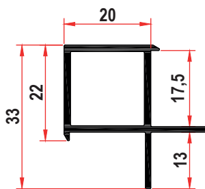
PRF-30062 0,400 Kg/m
