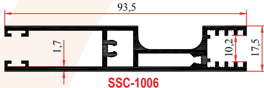
SSC-1006 1,220 Kg/m SÜRME ALT ETEK-10MM
