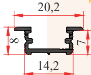
2905 G EKO 0,110 Kg/m
