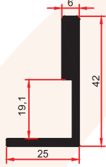
8755 0,615 Kg/m
