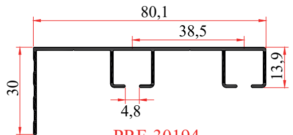
PRF-30194 0,495 Kg/m
