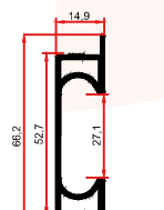
SM 1013 ÇT 0,530 Kg/m
