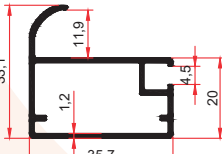
11383 A 0,455 Kg/m
