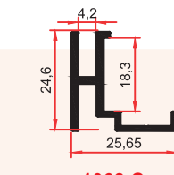
1068 G 0,335 Kg/m
