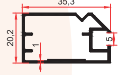
SM 1003 B 0,365 Kg/m
