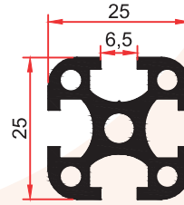
FS 4017 0,685 Kg/m
