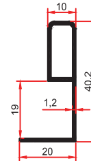
E-1436 0,300 Kg/m
