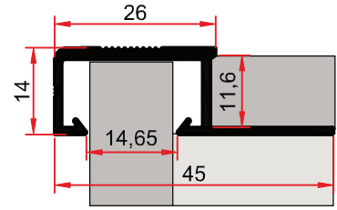
ST 253 A 0,289 kg/m Basamak Burunluğu STEPMOSE PROFILE
