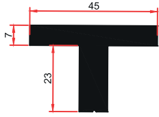
SM 6013 H 1,470 Kg/m
