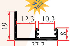
PRF-30429 0,215 Kg/m
