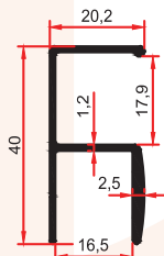
SM 1013 BF 0,365 Kg/m
