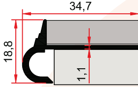
ST 253 C 0,216 kg/m Süslü Basamak Burunluğu STEPMOSE PROFILE
