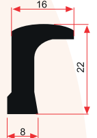
E 1986 0,485 Kg/m
