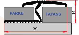
ST 206 0,240 kg/m
