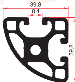
FS 4020 1,490 Kg/m
