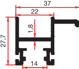
9007 B 0,483 kg/m
