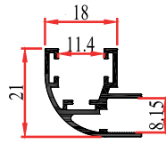
4249 CB - 0,210 Kg/m ALÜMİNYUM CAM H 8*10MM KÖŞE
