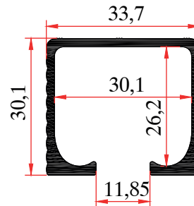
PRF-30278 0,575 Kg/m
