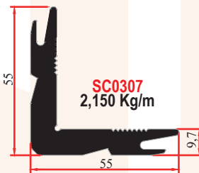
Köşe Birleştirme Aparatı
