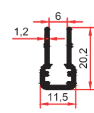
3211 0,190 Kg/m
