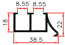
2108 0,385 Kg/m
