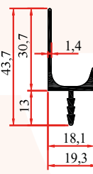
1013 ÇN EKO 0,350 Kg/m
