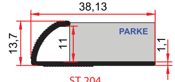
ST 204 0,192 kg/m
