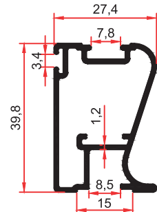
7344 0,550 Kg/m
