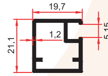
SM 1007 C 0,295 Kg/m
