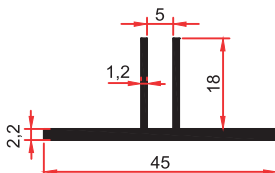
SM 1068 E 0,385 Kg/m
