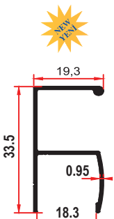
PRF-30523 0,225 Kg/m
