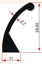
E 1077 0,435 Kg/m
