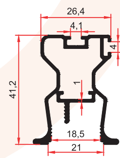
7473 0,520 Kg/m
