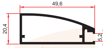
SM 1001 0,475 Kg/m
