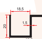
9435 0,335 Kg/m
