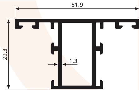
SD 1622 0,600 Kg/m
