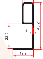
7574 0,265 Kg/m
