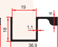
8781 0,295 Kg/m
