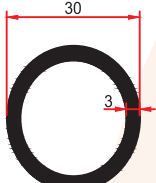
SM 5025 0,690 Kg/m
