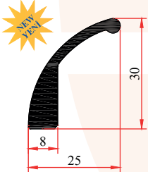
PRF-30165 0,465 Kg/m
