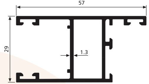
SD 1400 0,670 Kg/m
