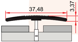
ST 217 0,213 kg/m
