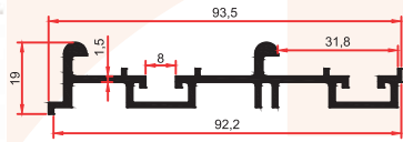
7691 A ÜST RAY 0,815 Kg/m
