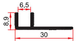
MP 45 0,172 kg/m
