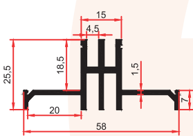
1068 C 0,640 Kg/m
