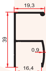
3796 A 0,235 Kg/m
