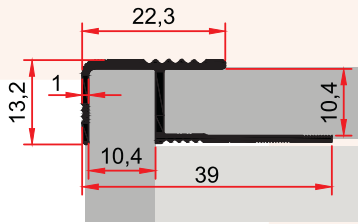
MP 20 0,207 kg/m
