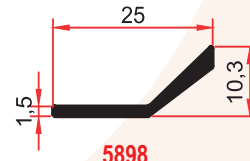
5898 0,125 Kg/m
