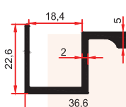
7505 0,410 Kg/m
