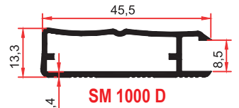
SM 1000 D 0,400 Kg/m
