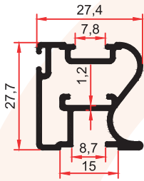
7345 0,470 Kg/m
