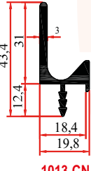
1013 ÇN 0,525 Kg/m
