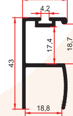
1013 BJ 0,435 Kg/m
