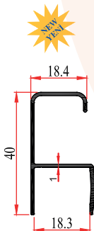
2527 EKO 0,290 Kg/m
