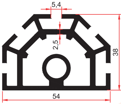
FS 4024 1,665 Kg/m
