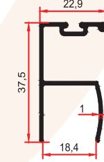
9476 0,295 Kg/m
