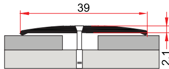
MP 7 0,172 kg/m
