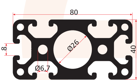
FS 4012 A 3,400 Kg/m
