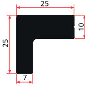
SM 6014 BK 1,005 Kg/m
