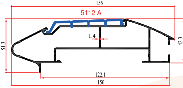
5112 A 1,730 Kg/m Yazar Kasa Tampon Profili
