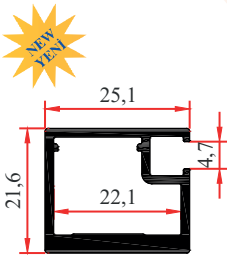
PRF-30407 0,490 Kg/m
