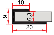
ST 215 0,124 kg/m
