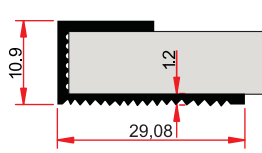
ST 225 A 0,144 kg/m
