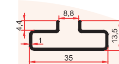
SM 1042 0,220 Kg/m
