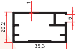
SM 1003 D 0,365 Kg/m
