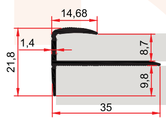
ST 246 E 0,227 kg/m
