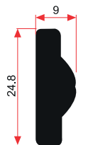
E 1175 0,465 Kg/m
