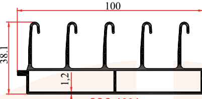
SSC-1001 1,410 Kg/m EŞİKLİ ALT RAY
