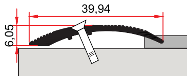
ST 230 A 0,213 kg/m
