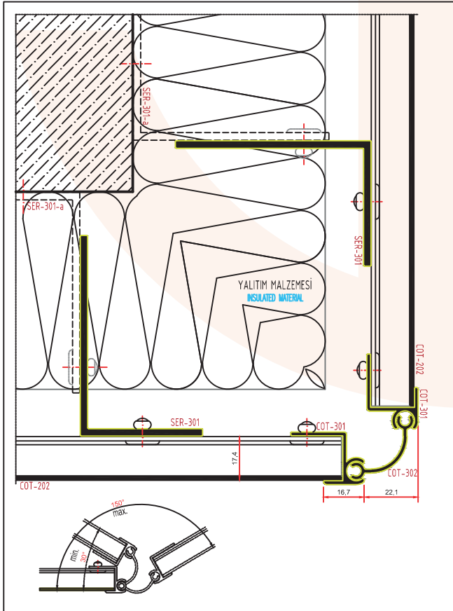
KÖŞE DETAY CORNER DETAIL
