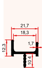
SM 1013 ÇK 0,220 Kg/m
