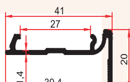
SM 1014 TL 0,290 Kg/m
