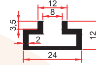
SM 1040 0,260 Kg/m
