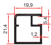
10954 0,275 Kg/m
