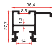
9007 E 0,440 kg/m (E Kulplu)
