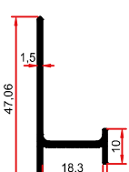
13440 A 0,305 Kg/m
