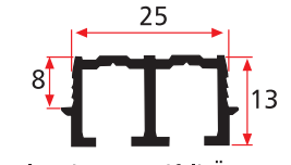
7615 Alüminyum Çiftli Üst Ray 0,265 Kg/m
