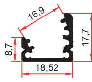
9028 0,180 Kg/m
