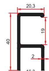
SM 1013 A 0,505 Kg/m
