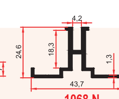
1068 N 0,425 Kg/m
