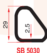
SB 5030 0,590 Kg/m
