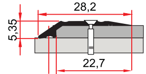
ST 242 0,113 kg/m
