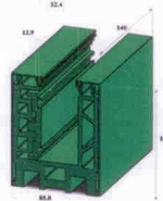
Şekil 1a 1.Küpeşte (2311,2312,2313)
