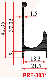
PRF-30319 0,505 Kg/m
