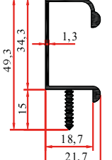
1013 CR 0,435 Kg/m
