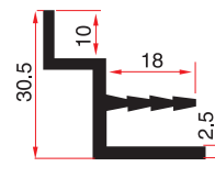
SM 1038 SA 0,485 Kg/m
