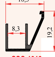
SSC-1013 0,165 Kg/m KENETLİ ÇONTA ALM-8MM
