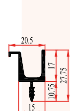
10548 0,290 Kg/m
