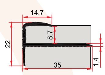
ST 246 C 0,227 kg/m
