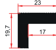
SM 6013 M 0,595 Kg/m
