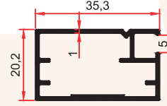
SM 1003 C 0,375 Kg/m
