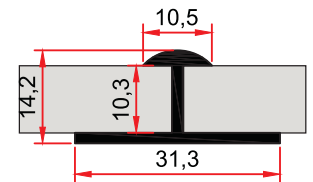
ST 232 0,227 kg/m
