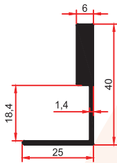
7503 0,485 Kg/m
