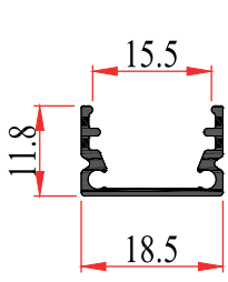
9029 0,140 Kg/m
