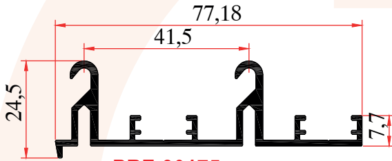
PRF-30175 0,790 Kg/m
