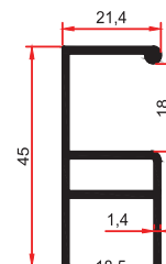
SM 1013 0,485 Kg/m
