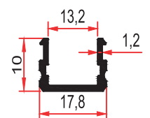
3714 0,125 Kg/m
