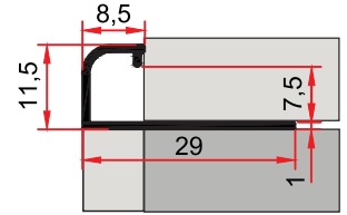
ST 248 A 0,128 kg/m 10 luk Fayans Çıtası 10 MM CERAMIC COVER PROFILE
