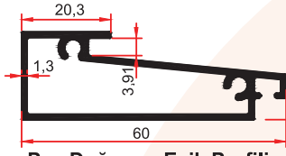
Pvc Doğrama Eşik Profili 8032 0,615 Kg/m
