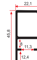
SM 1013 E 0,535 Kg/m
