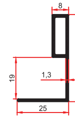
6536 0,335 Kg/m
