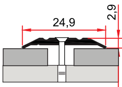
ST 243 0,097kg/m
