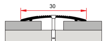
MP 31 0,090 kg/m
