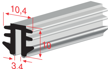
9477-1073 A ŞEFFAF U FİTİLİ
