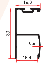
3797 A 0,255 Kg/m
