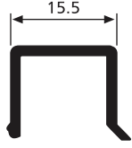
SD 1674 0,140 Kg/m
