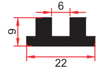
2112 0,340 Kg/m
