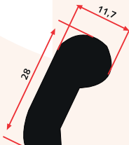
SM 6013 A 0,615 Kg/m
