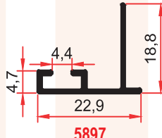
5897 0,110 Kg/m
