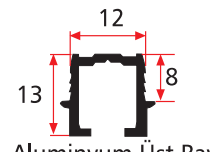
7610 Alüminyum Üst Ray 0,140 Kg/m
