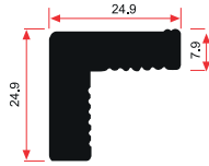
E 1391 0,880 Kg/m
