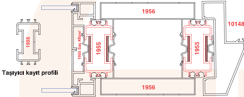
taban + kartlı geçiş sistemlerinde kapı yanı ve taban profili
