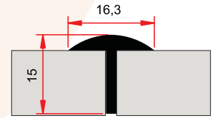
SM 1093 0,145 kg/m
