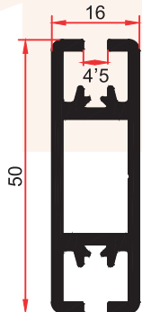
FS 4026 0,835 Kg/m
