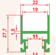
9007 A - PVC SİYAH BEYAZ GRİ
