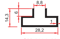
SM 1038 AL 0,195 Kg/m
