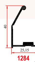
8669 0,455 Kg/m
