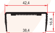
7628 0,285 Kg/m
