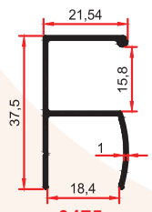
9475 0,265 Kg/m
