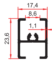
8062 0,255 Kg/m
