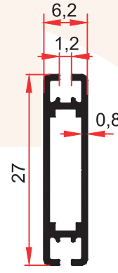
FS 4027 1,155 Kg/m
