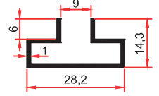
SM 1037 0,195 Kg/m
