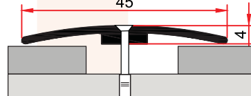
ST 226 A 0,248 kg/m
