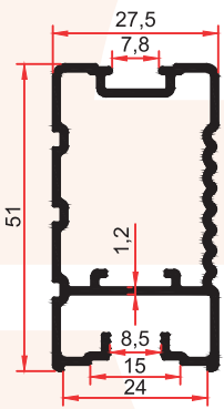
7349 0,655 Kg/m
