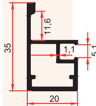
7356 0,365 Kg/m
