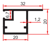
9741 0,315 Kg/m
