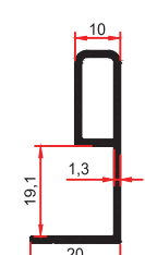
8756 0,325 Kg/m
