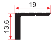
SM 1089 0,355 Kg/m
