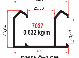
7027 0,632 kg/m
