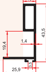
6622 0,405 Kg/m
