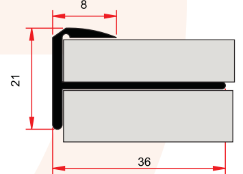
ST 246 0,250 kg/m
