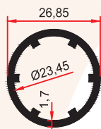
SM 5023 0,415 Kg/m
