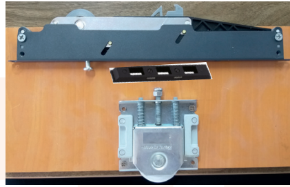
30097-3099 AHŞABA GÖRE MEKANİZMA SETİ
