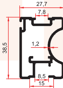
7346 0,565 Kg/m
