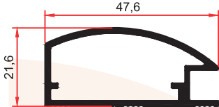
SM 1001 D 0,535 Kg/m
