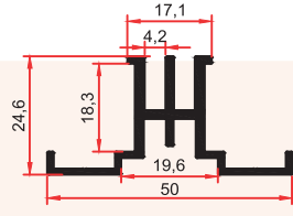
1068 F 0,525 Kg/m
