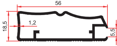
SM 1000 B 0,545 Kg/m
