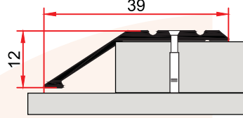
MP 29 0,169 kg/m
