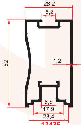
13436 0,625 Kg/m
