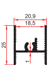
7475 0,245 Kg/m
