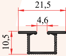
PRF-30097 0,135 Kg/m
