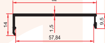
SM 1015 0,325 Kg/m
