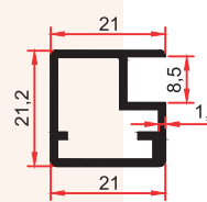
SM 1007 N 0,305 Kg/m
