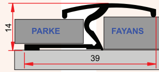
ST 205 0,270 kg/m
