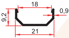
3298 0,085 Kg/m 9029 ALM KLİPS
