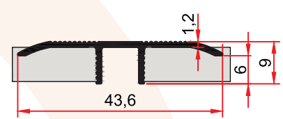
ST 212 E 0,180 kg/m
