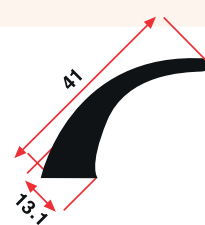
SM 6013 C 0,645 Kg/m
