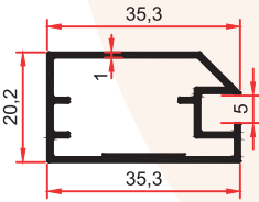
SM 1003 A 0,365 Kg/m
