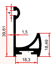
8580 0,500 Kg/m
