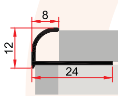
ST 248 C 0,105 kg/m 10 luk Fayans Çıtası 10 MM CERAMIC COVER PROFILE
