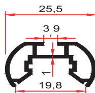
9030 0,265 Kg/m
