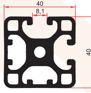
FS 4014 1,825 Kg/m
