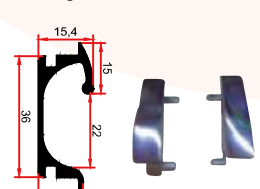
E 1228 0,390 Kg/m
