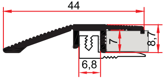
ST 230 0,248 kg/m
