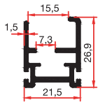
7005 F 0,402 kg/m (Isıcamlı Kanat)
