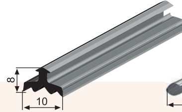
3000-3002 BASKI ÇİTA FİTİLİ
