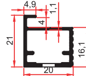
SM 1007 E 0,275 Kg/m
