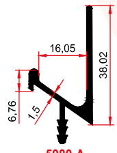
5980 A 0,410 Kg/m
