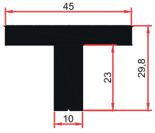
SM 6013 I 1,425 Kg/m
