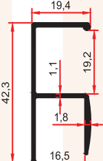
6066 0,305 Kg/m
