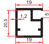
SM 1007 0,275 Kg/m
