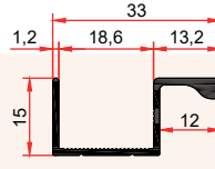
9382 0,230 Kg/m
