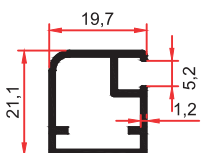
SM 1007 D 0,285 Kg/m
