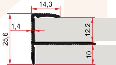
ST 246 D 0,290 kg/m
