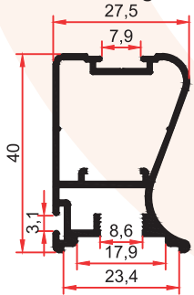
13431 0,515 Kg/m
