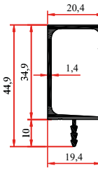
SM 1013 G EKO 0,380 Kg/m
