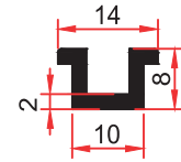
SM 1097 0,140 Kg/m
