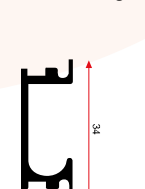
E 1659 0,320 Kg/m
