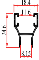
4825 CB - 0,210 Kg/m ALÜMİNYUM CAM H 8*10MM
