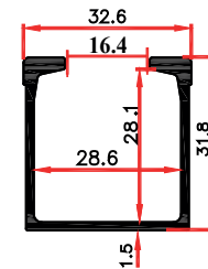
PRF-30219 0,490 Kg/m
