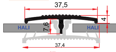
ST 212 0,205 kg/m
