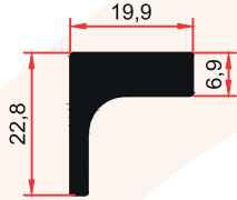
E 1304 0,510 Kg/m
