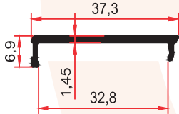
SM 1014 TY 0,175 Kg/m
