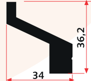
SM 6013 J 0,980 Kg/m
