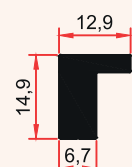
E 1014 0,320 Kg/m
