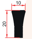
SM 6013 K 0,375 Kg/m
