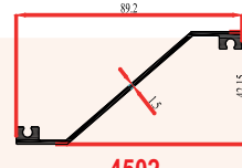
4502 0,600 Kg/m
