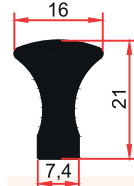
E 1657 0,475 Kg/m
