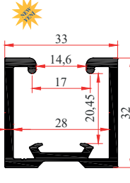
PRF-30495 0,790 Kg/m
