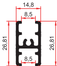
5167 0,320 Kg/m
