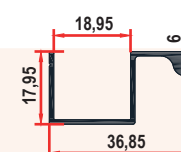
7505 EKO 0,290 Kg/m
