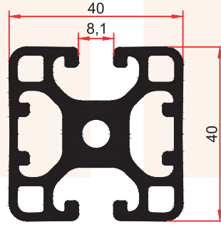
FS 4013 1,825 Kg/m
