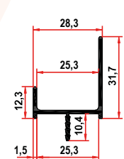
PRF-30168 0,320 Kg/m
