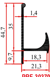
PRF-30370 0,360 Kg/m
