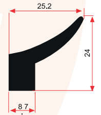
E 1656 0,520 Kg/m
