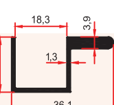
7405 0,345 Kg/m
