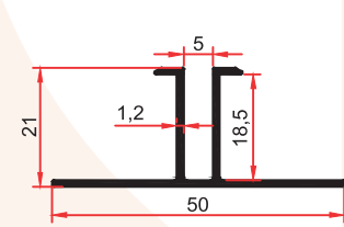
1068 D 0,315 Kg/m
