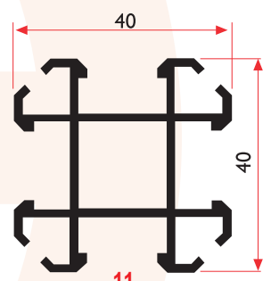
FS 4018 0,940 Kg/m
