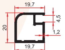
SM 1007 F 0,265 Kg/m
