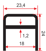
SM 1012 0,410 Kg/m
