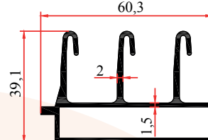
SSC-1004 1,070 Kg/m EŞİKLİ ALT RAY
