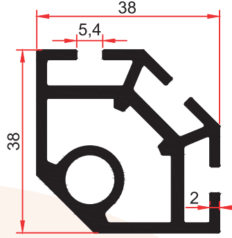
FS 4025 1,210 Kg/m
