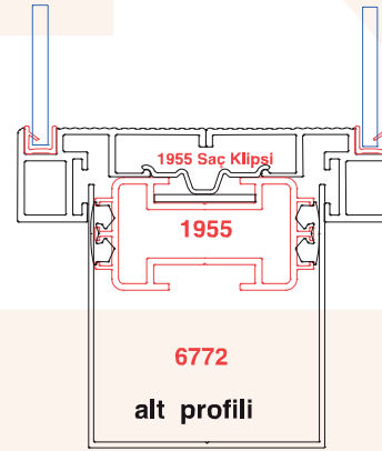
taban + kartlı geçiş sistemlerinde kapı yanı ve taban profili
