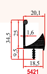
5421 0,485 Kg/m
