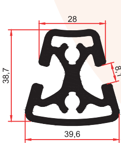
FS 4019 1,655 Kg/m
