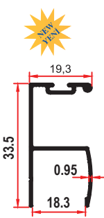
PRF-30524 0,245 Kg/m
