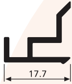
SD 1410 0,150 Kg/m
