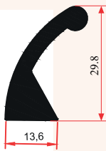
SM 6013 F 0,605 Kg/m
