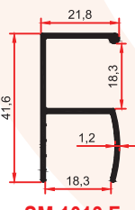
SM 1013 F 0,335 Kg/m
