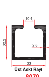
8079 0,850 Kg/m
