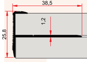
ST 246 A 0,210 kg/m
