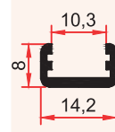
2905 0,115 Kg/m
