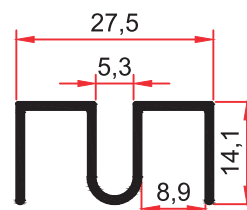
7308 0,225 Kg/m
