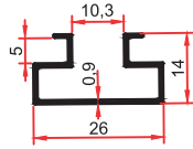
8585 0,175 Kg/m
