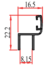
4166 CB - 0,175 Kg/m ALÜMİNYUM CAM H 8MM
