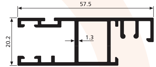
SD 1401 0,700 Kg/m
