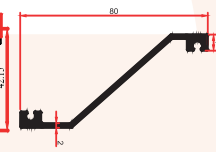
6014 A 0,685 Kg/m
