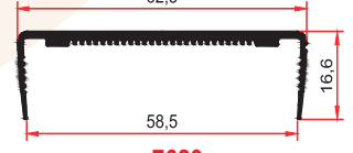
7629 0,395 Kg/m
