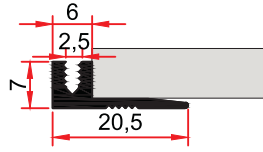
ST 231 0,130 kg/m
