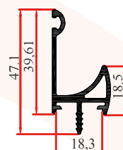
8580 A 0,510 Kg/m
