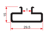
SM 1045 A 0,315 Kg/m
