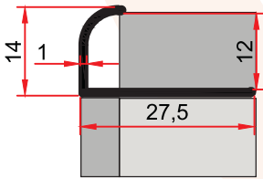
MP 25 0,119 kg/m
