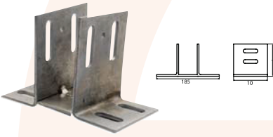
U Tipi Cephe Ankraji U Type Facade Anchor
