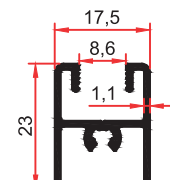
6830 0,265 Kg/m
