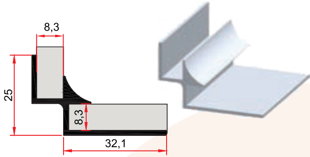
ST 229 A 0,340 kg/m
