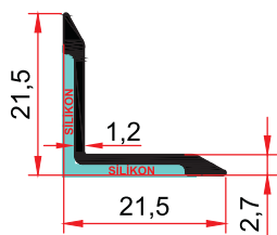
MP 15 0,146 kg/m
