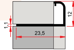
ST 250 A 0,115 kg/m 12 lik Fayans Çıtası 12 MM CERAMIC COVER PROFILE
