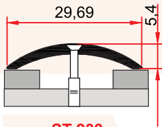
ST 239 0,154 kg/m
