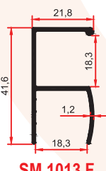
SM 1013 F 0,335 Kg/m
