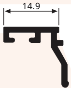
SD 1376 0,165 Kg/m
