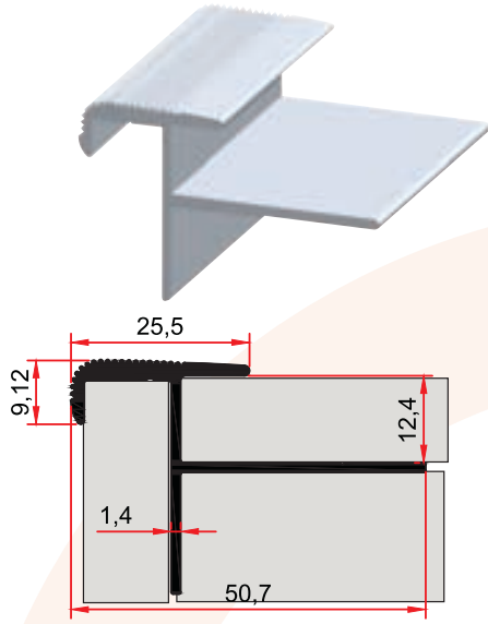
ST 229 B 0,419 kg/m
