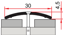
ST 239 A 0,132 kg/m
