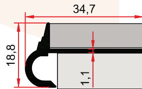
ST 253 C 0,216 kg/m Süslü Basamak Burunluđu STEPNOSE PROFILE
