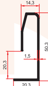
SM 1013 Y 0,425 Kg/m
