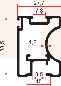
7346 0,565 Kg/m
