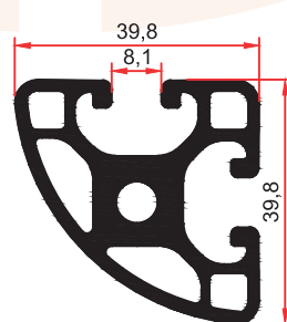
FS 4020 1,490 Kg/m
