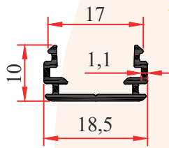
PRF-30400 0,130 Kg/m
