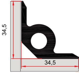
SM 2011 0,926 kg/m
