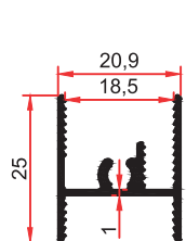
7475 0,245 Kg/m
