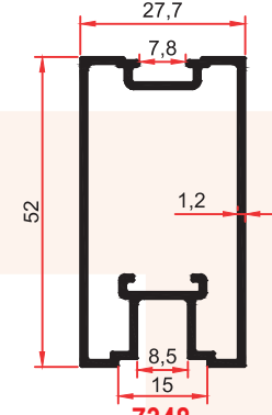
7348 0,645 Kg/m
