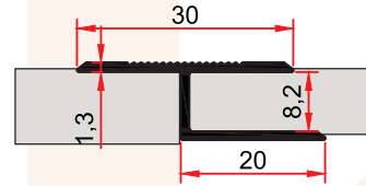
ST 245 0,186 kg/m
