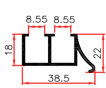
2108 0,385 Kg/m
