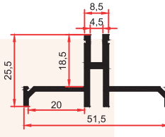
1068 H 0,495 Kg/m
