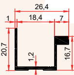
1936 0,240 Kg/m
