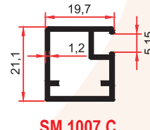
SM 1007 C 0,295 Kg/m
