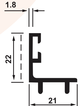
SD 2133 0,315 Kg/m
