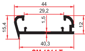
SM 1014 T 0,330 Kg/m
