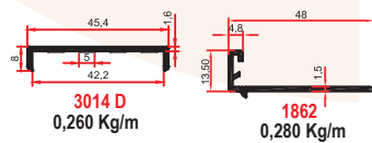
LAMİNAT ÇİFT KAPI ADAPTÖRÜ
