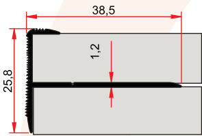
ST 246 A 0,210 kg/m
