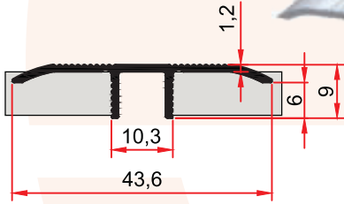
ST 212 E 0,180 kg/m
