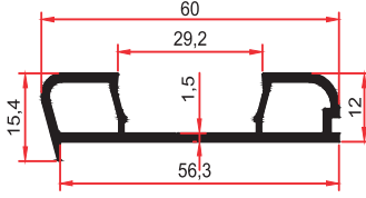
SM 1014 T6 0,485 Kg/m
