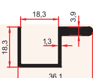
7405 0,345 Kg/m
