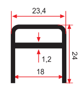
SM 1012 0,410 Kg/m
