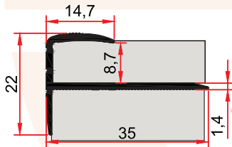
ST 246 C 0,227 kg/m
