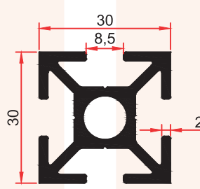
FS 4016 A 0,925 Kg/m
