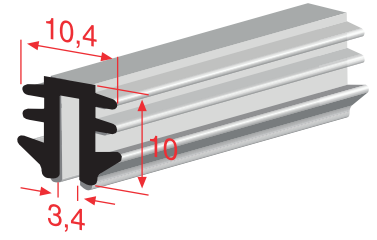
9477-1073 A ŞEFAF U FİTİLİ
