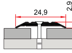
ST 243 0,097 kg/m
