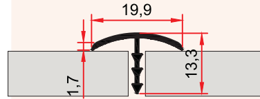
SM 1023 A 0,092 kg/m
