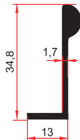
SM 1082 B 0,300 Kg/m
