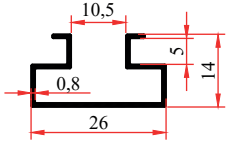
4301 0,160 Kg/m
