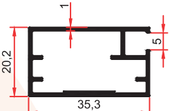
SM 1003 D 0,365 Kg/m
