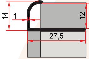
MP 25 0,119 kg/m
