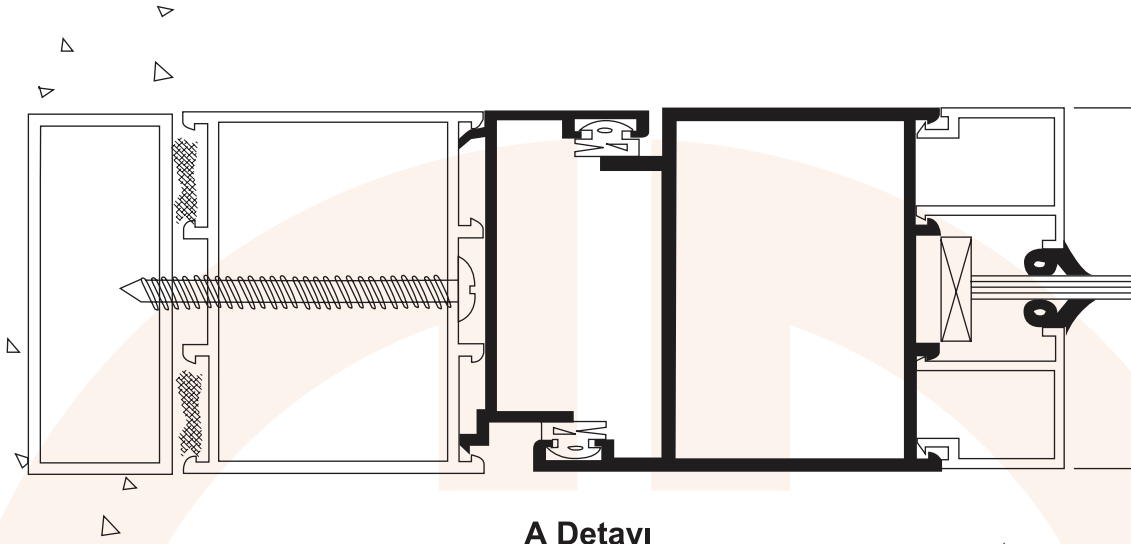
A Detayı
