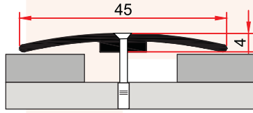
ST 226 A 0,248 kg/m
