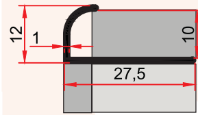
MP 26 0,114 kg/m
