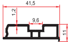
SM 1014 TN 0,350 Kg/m
