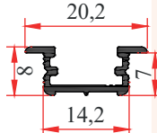
2905 G EKO 0,110 Kg/m
