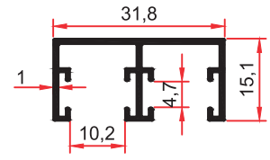
2109 A 0,265 Kg/m
