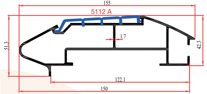
5112 B 2,040 Kg/m Yazar Kasa Tampon Profili
