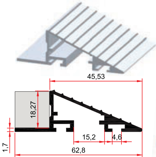
ST 230 R 0,552 kg/m
