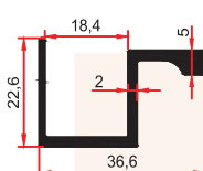
7505 0,410 Kg/m
