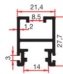
9007 D 0,440 kg/m (D Kulpsuz)
