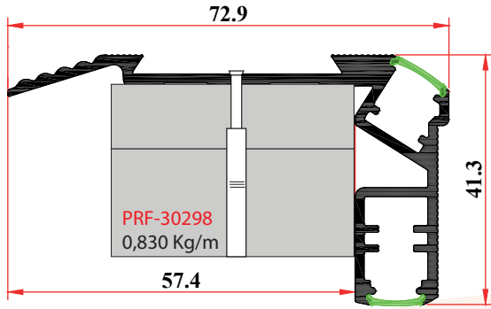
12252 / PRF-30298 BASAMAK PRF KAPAĞI
