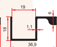
8781 0,295 Kg/m
