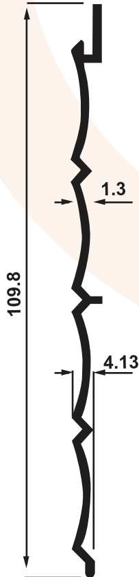
SD 2874 0,455 Kg/m
