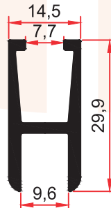
7309 0,410 Kg/m
