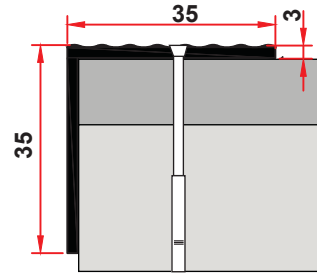
PRF-30475 0,505 kg/m
