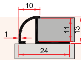
ST 248 F 0,130 kg/m
