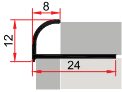
ST 248 C 0,105 kg/m 10 luk Fayans Çıtası 10 MM CERAMIC COVER PROFILE
