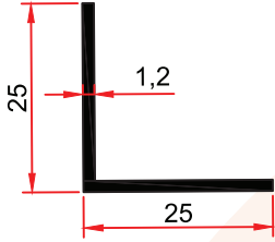
ST 236 0,158 kg/m
