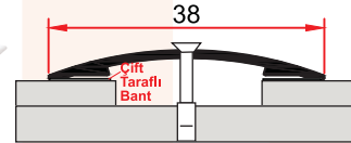
ST 239 C 0,132 kg/m
