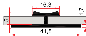
ST 232 A 0,308 kg/m
