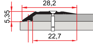
ST 242 0,113 kg/m
