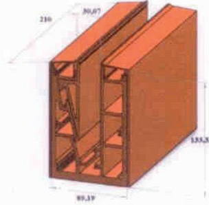
Şekil 1b 2.Küpeşte (11153,11152,11151)
