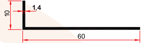
9458 0,260 kg/m
