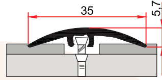
ST 227 0,186 kg/m
