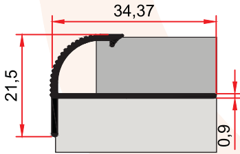
ST 255 0,184 kg/m Basamak Burunluğu STEPMOSE PROFILE
