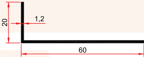
ST 238 0,255 kg/m
