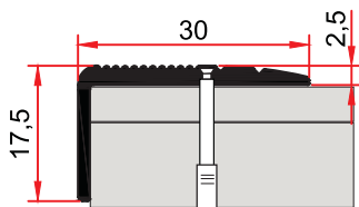
MP 40 0,232 kg/m
