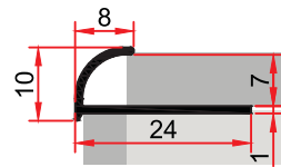
ST 248 B 0,100 kg/m 8 lik Fayans Çıtası 8 MM CERAMIC COVER PROFILE
