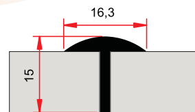
SM 1093 0,145 kg/m
