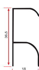
E 1910 0,225 Kg/m
