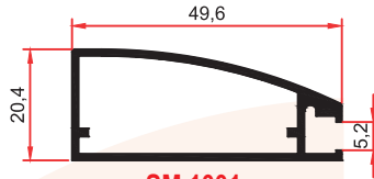
SM 1001 0,475 Kg/m
