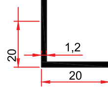
ST 235 0,124 kg/m
