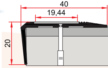
MP 35 0,246 kg/m
