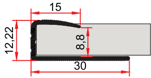
ST 214 0,168 kg/m
