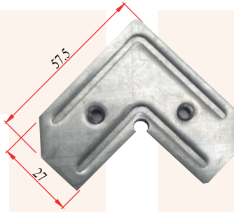
9896 SAÇ KÖŞE
