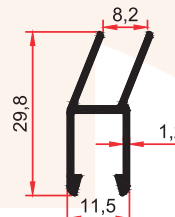
2110 B 0,240 Kg/m
