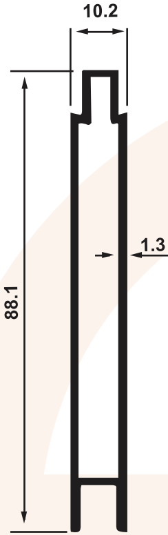
SD 1249 0,690 Kg/m
