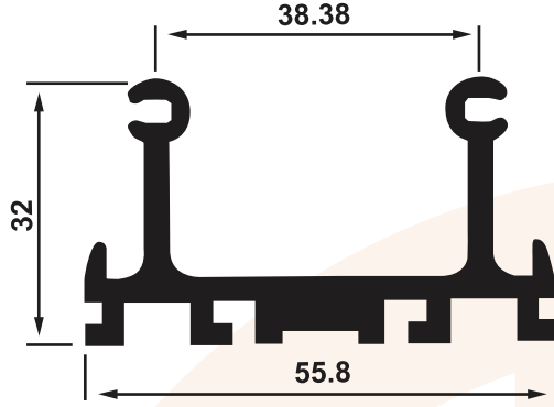
SD 2131 1,320 Kg/m S-60 Orta Bağlantı Profili
