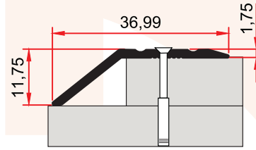
ST 241 C 0,171 kg/m
