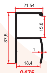
9475 0,265 Kg/m
