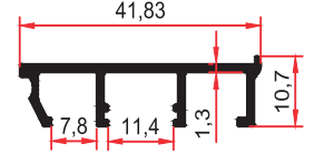
6236 0,285 Kg/m
