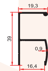
3796 A 0,235 Kg/m
