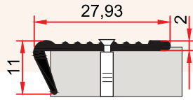
MP 51 0,154 kg/m
