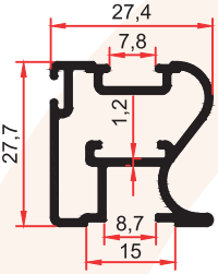
7345 0,470 Kg/m
