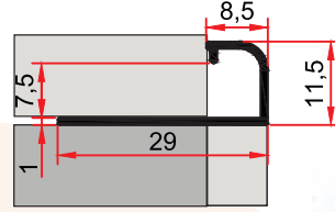
ST 248 A 0,128 kg/m 10 luk Fayans Çıtası 10 MM CERAMIC COVER PROFILE
