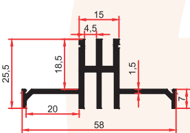
1068 C 0,640 Kg/m
