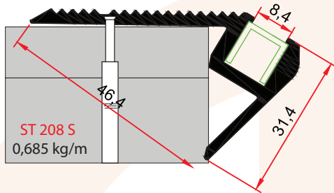
ST 208 S Led Kapağı
