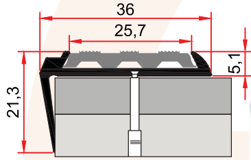
MP 36 0,246 kg/m
