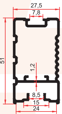
7349 0,655 Kg/m
