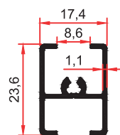
8062 0,255 Kg/m
