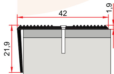
ST 244 0,231 kg/m
