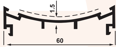
SD 1555 0,480 Kg/m
