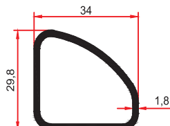
SB 5030 A 0,500 Kg/m
