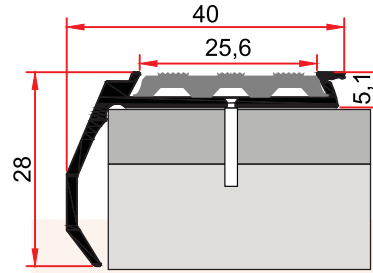
MP 37 0,286 kg/m
