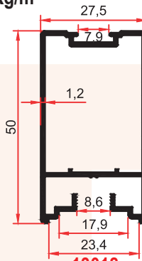
13018 0,570 Kg/m
