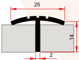
SM 1023 0,188 kg/m
