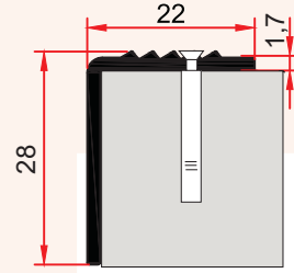
MP 48 0,228 kg/m
