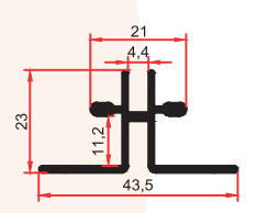
1068 B 0,410 Kg/m
