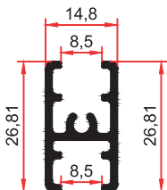
5167 0,320 Kg/m
