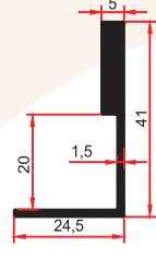
9126 A 0,445 Kg/m
