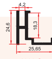
1068 G 0,335 Kg/m
