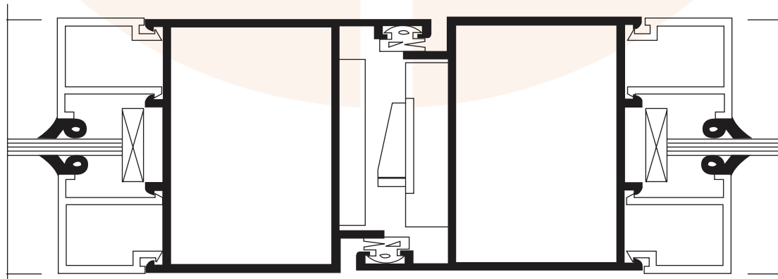
C Detayı
