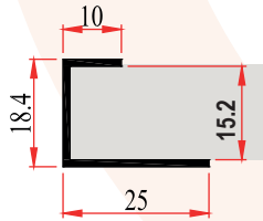
ST 228 A 0,215 kg/m
