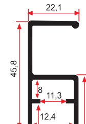
SM 1013 E 0,535 Kg/m
