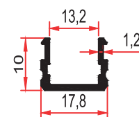
3714 0,125 Kg/m
