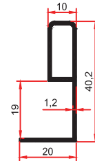
E-1436 0,300 Kg/m
