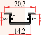
2905 G 0,130 Kg/m
