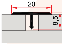
SM 1022 A 0,084 kg/m
