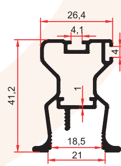
7473 0,520 Kg/m
