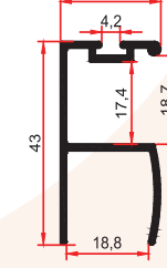
1013 BJ 0,435 Kg/m
