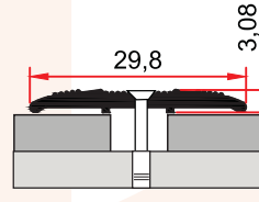
ST 243 A 0,155 kg/m
