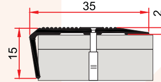
MP 39 0,180 kg/m
