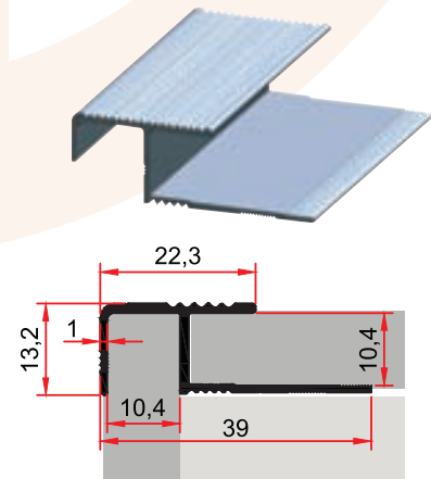
MP 20 0,207 kg/m
