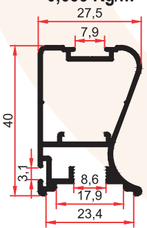
13431 0,515 Kg/m
