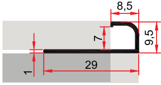
ST 248 0,119 kg/m 8 lik Fayans Çıtası 8 MM CERAMIC COVER PROFILE
