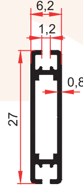
FS 4027 1,155 Kg/m
