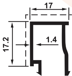
SD 2123 0,250 Kg/m
