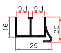
2108 M 0,290 Kg/m
