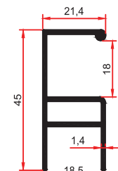
SM 1013 0,485 Kg/m
