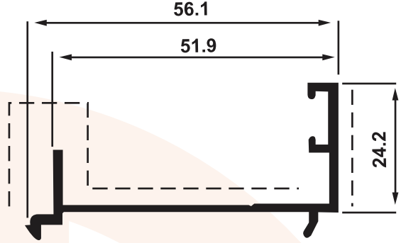
SD 1415 0,510 Kg/m
