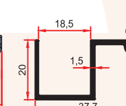
9435 0,335 Kg/m
