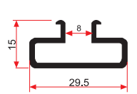
SM 1045 A 0,315 Kg/m
