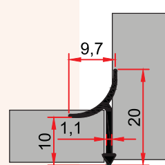
MP 28 0,079 kg/m
