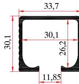
PRF-30278 0,575 Kg/m
