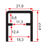
SM 1012 A 0,350 Kg/m
