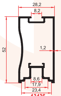
13436 0,625 Kg/m
