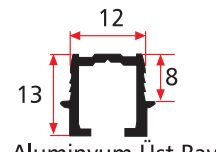
7610 Alüminyum Üst Ray 0,140 Kg/m
