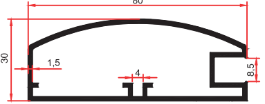
SM 1001 C 0,955 Kg/m
