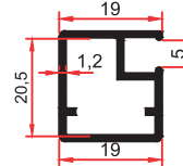
SM 1007 0,275 Kg/m
