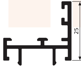
SD 1375 0,375 Kg/m
