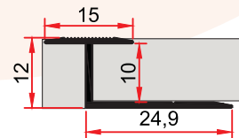
MP 30 0,125 kg/m
