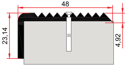
MP 47 0,660 kg/m
