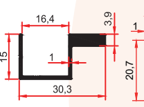
8965 0,255 Kg/m
