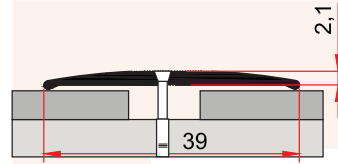
MP 7 0,172 kg/m
