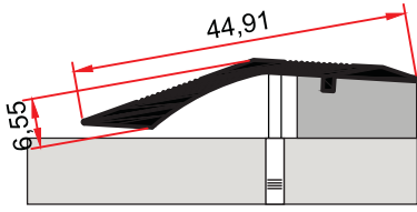
ST 230 B 0,234 kg/m
