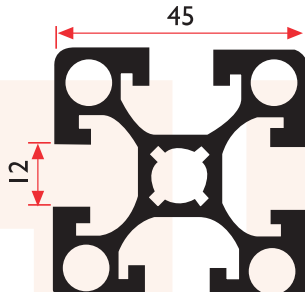
FS 4012 B 2,065 Kg/m
