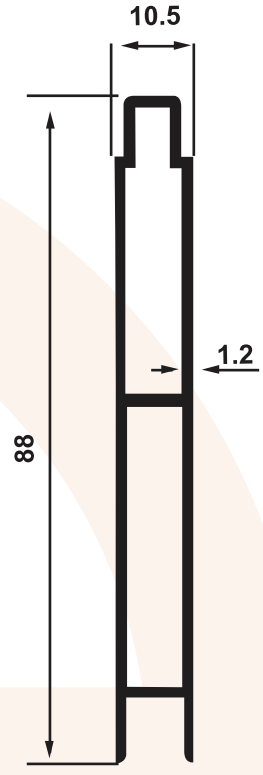
SD 4647 0,650 Kg/m
