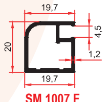
SM 1007 F 0,265 Kg/m
