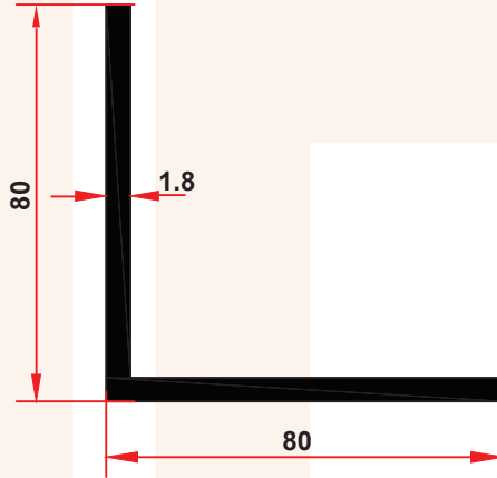
7249 0,770 kg/m
