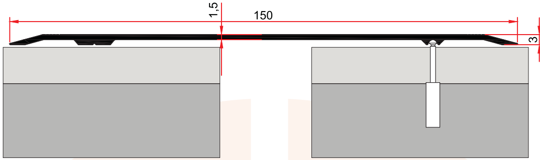
ST 247 F 0,650 kg/m
