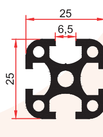
FS 4017 0,685 Kg/m
