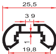
9030 0,265 Kg/m
