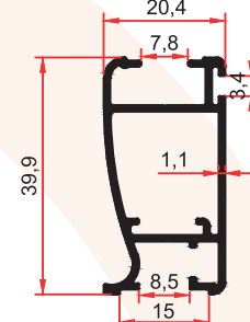
7347 0,430 Kg/m
