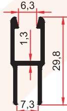
2110 A 0,235 Kg/m
