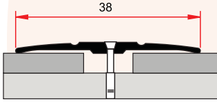
MP 6 0,137 kg/m
