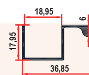
7505 EKO 0,290 Kg/m
