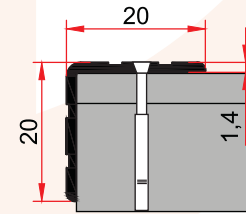
MP 19 0,140 kg/m
