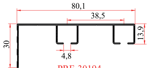
PRF-30194 0,495 Kg/m
