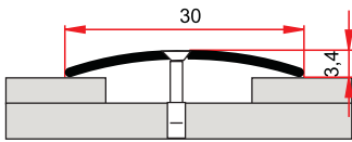
ST 239 E 0,090 kg/m
