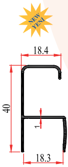
2527 EKO 0,290 Kg/m
