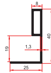
6536 0,335 Kg/m
