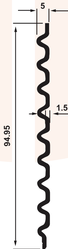
SD 4536 0,510 Kg/m
