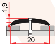
MP 5 0,097 kg/m
