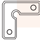
SM 1007 D SAÇ KÖŞE
