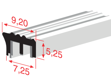
AYNA FİTİLİ
