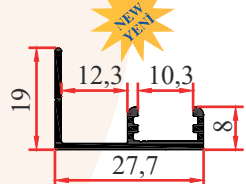
PRF-30429 0,215 Kg/m
