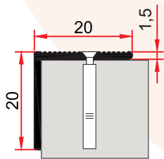
MP 49 0,146 kg/m
