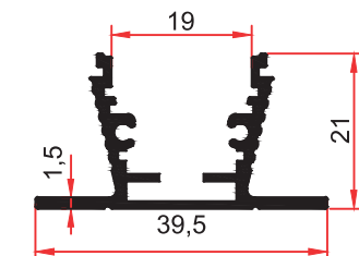
3735 0,375 Kg/m
