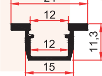
8607 0,165 Kg/m
