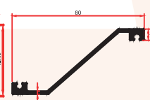
6014 A 0,685 Kg/m
