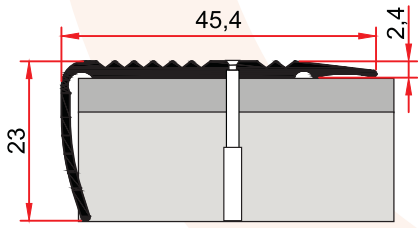
MP 38 0,284 kg/m
