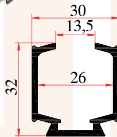
PRF-30140 0,565 Kg/m
