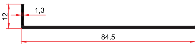
SM 1064 D 0,335 kg/m
