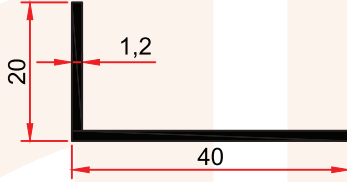
ST 237 0,192 kg/m
