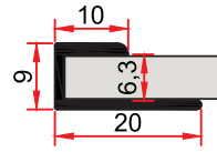
ST 215 0,124 kg/m
