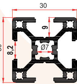
FS 4016 0,835 Kg/m
