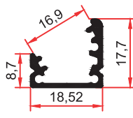
9028 0,180 Kg/m
