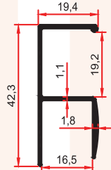
6066 0,305 Kg/m
