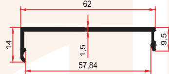
SM 1015 0,325 Kg/m
