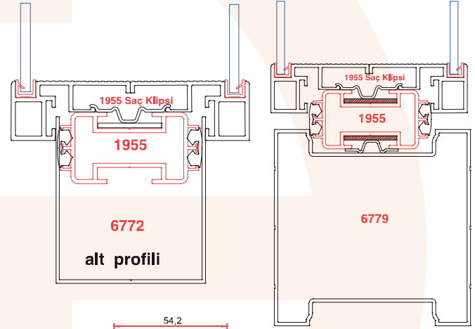
taban + kartlı geçiş sistemlerinde kapı yanı ve taban profili
