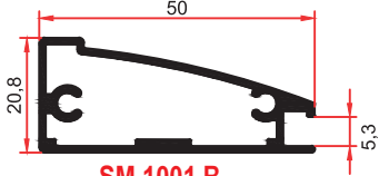
SM 1001 B 0,570 Kg/m
