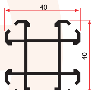
FS 4018 0,940 Kg/m
