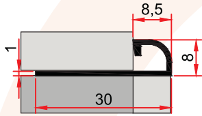
ST 249 0,130 kg/m 6'lık Fayans Çıtası 6 MM CERAMIC COVER PROFILE
