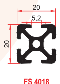
FS 4018 0,465 Kg/m
