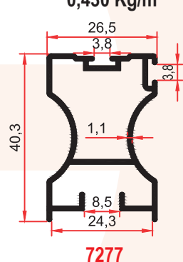
7277 0,480 Kg/m
