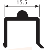
SD 1377 0,190 Kg/m
