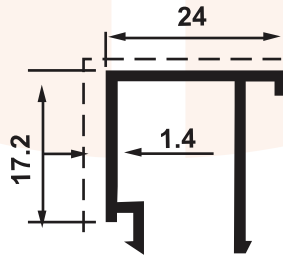
SD 1416 0,280 Kg/m
