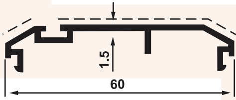
SD 1554 0,500 Kg/m
