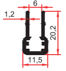
3211 0,190 Kg/m
