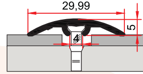
MP 5 0,140 kg/m
