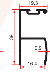
3797 A 0,255 Kg/m
