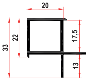
PRF-30062 0,400 Kg/m
