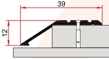
MP 29 0,169 kg/m
