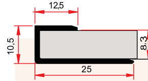
ST 228 0,135 kg/m
