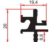
SM 1038 B 0,415 Kg/m
