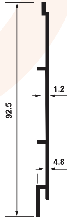
SD 1317 0,360 Kg/m
