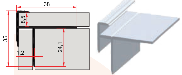
ST 229 0,275 kg/m
