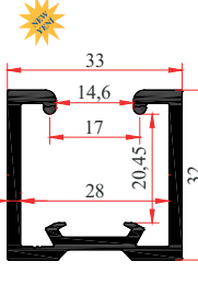
PRF-30495 0,790 Kg/m
