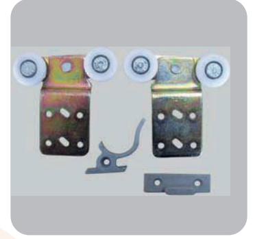
SKM 38 YL-R SÜTLÜK RULMANI ÇİFTİ
