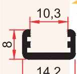
2905 0,115 Kg/m
