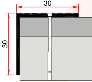
MP 21 0,252 kg/m
