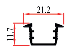
6798 0,140 Kg/m
