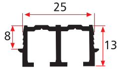
7615 Alüminyum Çiftli Üst Ray 0,265 Kg/m
