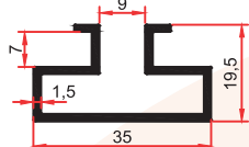
SM 1045 0,410 Kg/m
