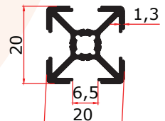
FS 4013 H 0,345 Kg/m
