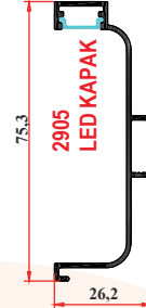
LEDLİ GİZLİ KULP 2676 L 0,460 Kg/m
