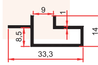
SM 1043 0,195 Kg/m
