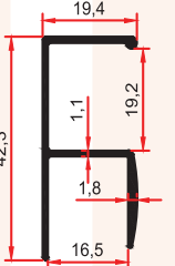
6066 0,305 Kg/m
