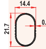
12050 0,120 Kg/m
