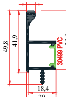
PRF-30612 0,490 Kg/m
