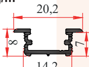
2905 G EKO 0,110 Kg/m
