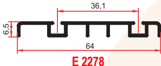
E 2278 0,355 Kg/m
