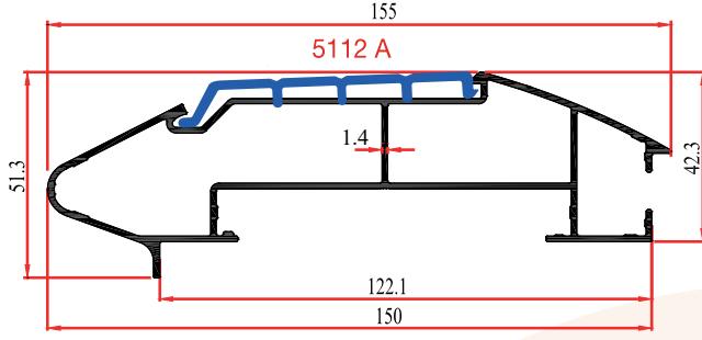
5112 B EKO Yazar Kasa Tampon Profili 1,730 Kg/m
