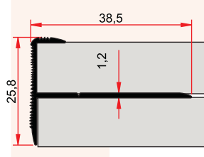
ST 246 A 0,210 kg/m
