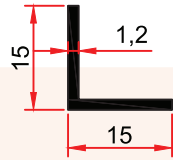
ST 234 0,093 kg/m
