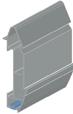
5112 Yazar Kasa Tampon Profili 3,245 Kg/m
