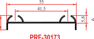
PRF-30173 0,225 Kg/m
