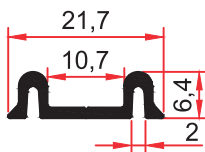
7307 0,140 Kg/m
