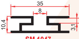
SM 1047 0,295 Kg/m
