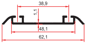
5677 0,270 Kg/m
