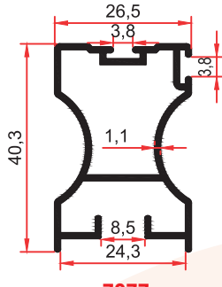
7277 0,480 Kg/m
