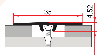
ST 227 B 0,130 kg/m
