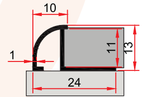
ST 248 F 0,130 kg/m
