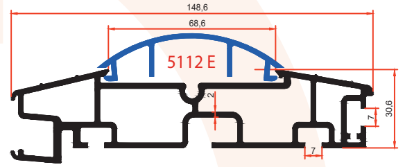
5112 E Yazar Kasa Tampon Profili 2,824 Kg/m
