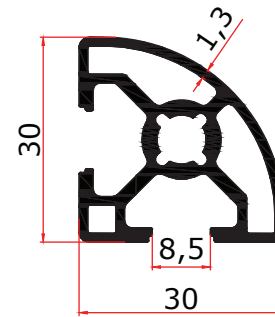
FS 4013 G 0,675 Kg/m
