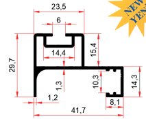
PRF-30672 0,497 Kg/m
