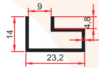
SM 1046 0,165 Kg/m
