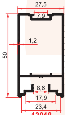
13018 0,570 Kg/m
