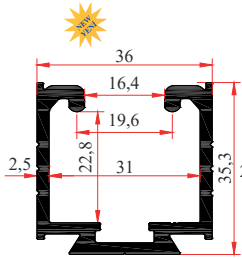
PRF-30490 0,890 Kg/m
