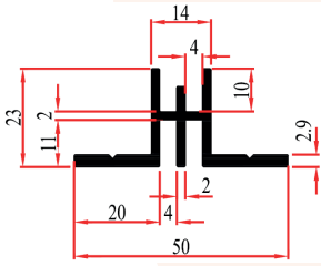
S-GNC ÇİFTLİ TİJ BOY 300CM 0,710 Kg/m 12 MM HATVELİ
