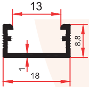
3064 0,105 Kg/m
