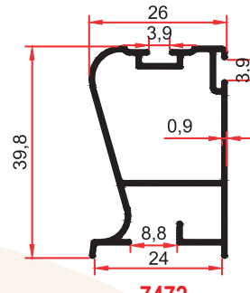
7472 0,375 Kg/m
