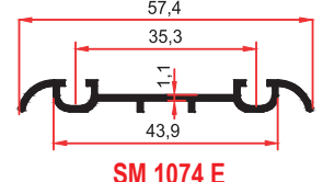
SM 1074 E 0,245 Kg/m
