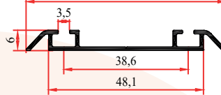
SM 1074 B 0,325 Kg/m
