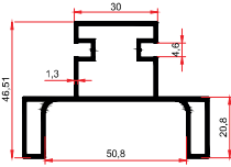
12387 A 0,890 Kg/m
