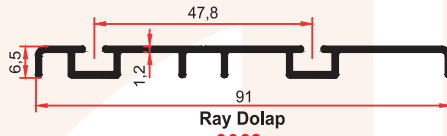
Ray Dolap 9068 0,455 Kg/m
