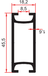
FS 4032 0,580 Kg/m
