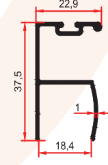
9476 0,295 Kg/m
