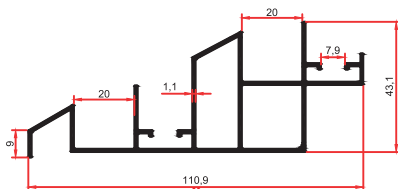
7689 ÜST RAY 1,005 Kg/m
