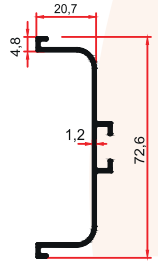
2676 A 0,415 Kg/m
