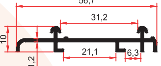
SM 1074 0,315 Kg/m
