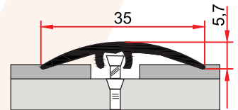
ST 227 0,186 kg/m
