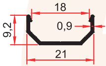
3298 0,085 Kg/m 9029 ALM KLİPS
