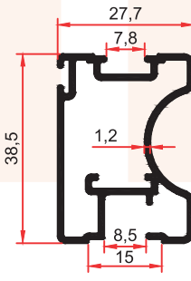
7346 0,565 Kg/m
