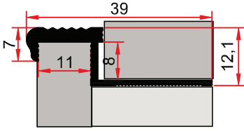
ST 253 D 0,173 kg/m Basamak Burunluğu STEPPED PROFILE
