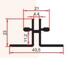
1068 B 0,410 Kg/m
