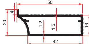
7352 C 0,445 Kg/m
