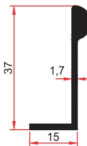
SM 1082 C 0,320 Kg/m
