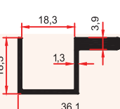
7405 0,345 Kg/m
