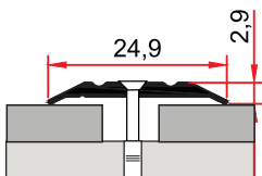
ST 243 0,097kg/m
