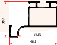
4470 0,560 Kg/m
