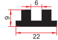
2112 0,340 Kg/m
