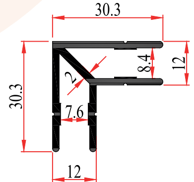
SD 1671 0,555 Kg/m
