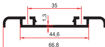
5169 0,365 Kg/m
