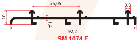
SM 1074 F 0,590 Kg/m
