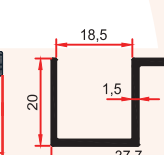
9435 0,335 Kg/m
