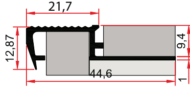
ST 253 0,257 kg/m Basamak Burunluğu STEPPED PROFILE
