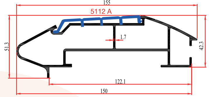
5112 B Yazar Kasa Tampon Profili 2,040 Kg/m
