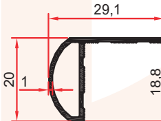
4746 0,185 Kg/m
