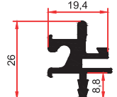
SM 1038 B 0,415 Kg/m
