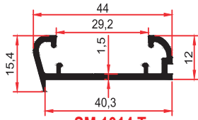
SM 1014 T 0,330 Kg/m
