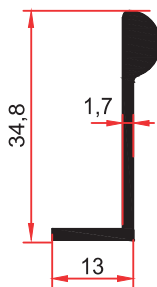
SM 1082 B 0,300 Kg/m
