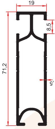
FS 4030 0,790 Kg/m
