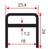
SM 1012 0,410 Kg/m
