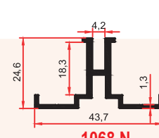
1068 N 0,425 Kg/m
