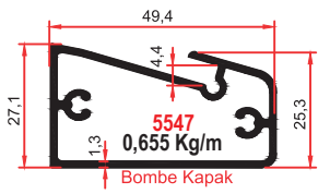
5547 Bombe Kapak 0,655 Kg/m
