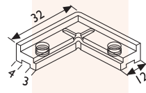
SM 1005 ZAMAK KÖŞE
