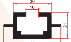
SM 1047 A 0,760 Kg/m
