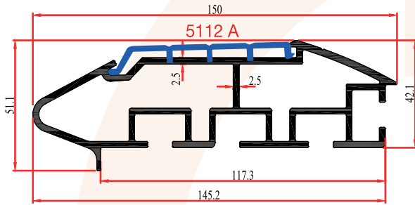
5112 Yazar Kasa Tampon Profili 3,245 Kg/m
