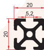
FS 4018 0,465 Kg/m
