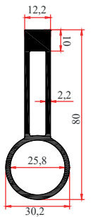
PRF-30538 1,340 Kg/m 25*1 MM BORU PRF-30576 ASKI TUTUCUSU
