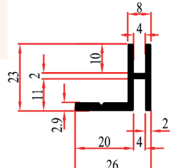
S-GNC TEKİLİ TİJ BOY 300CM 0,410 Kg/m 12 MM HATVELİ
