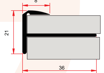
ST 246 0,250 kg/m
