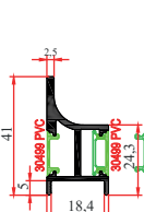
PRF-30547 0,480 Kg/m
