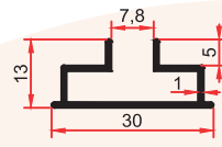
SM 1041 0,190 Kg/m
