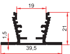
3735 0,375 Kg/m
