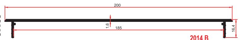
2014 B 0,975 Kg/m
