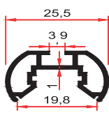
9030 0,265 Kg/m
