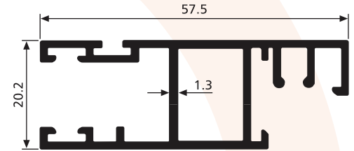
SD 1401 0,700 Kg/m
