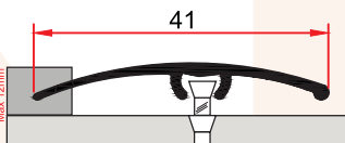
ST 227 A 0,154 kg/m
