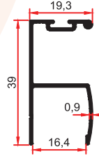
3797 A 0,255 Kg/m
