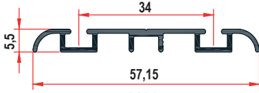
2196 0,280 Kg/m
