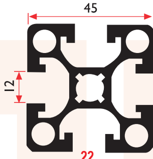
22 1,820 Kg/m
