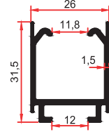
SM 1092 A 0,424 Kg/m
