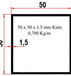
50x50 ROTİL AYAK
