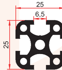
FS 4017 0,685 Kg/m
