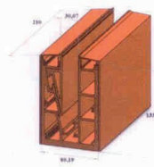
Şekil 1b 2.Küpeşte (11153,11152,11151)
