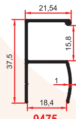
9475 0,265 Kg/m
