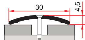
ST 239 A 0,132 kg/m
