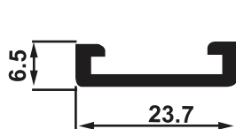
SD 1145 0,205 Kg/m
