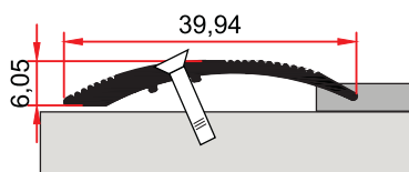
ST 230 A 0,213 kg/m
