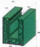
Şekil 1a 1.Küpeşte (2311,2312,2313)
