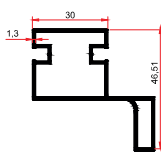
12388 A 0,670 Kg/m
