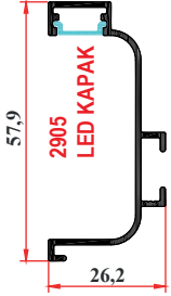
LEDLİ GİZLİ KULP 2675 L 0,400 Kg/m
