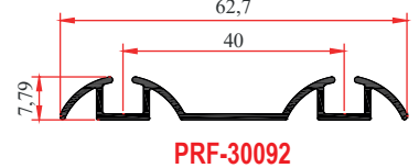
PRF-30092 0,315 KG/M
