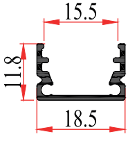
9029 EKO 0,115 Kg/m
